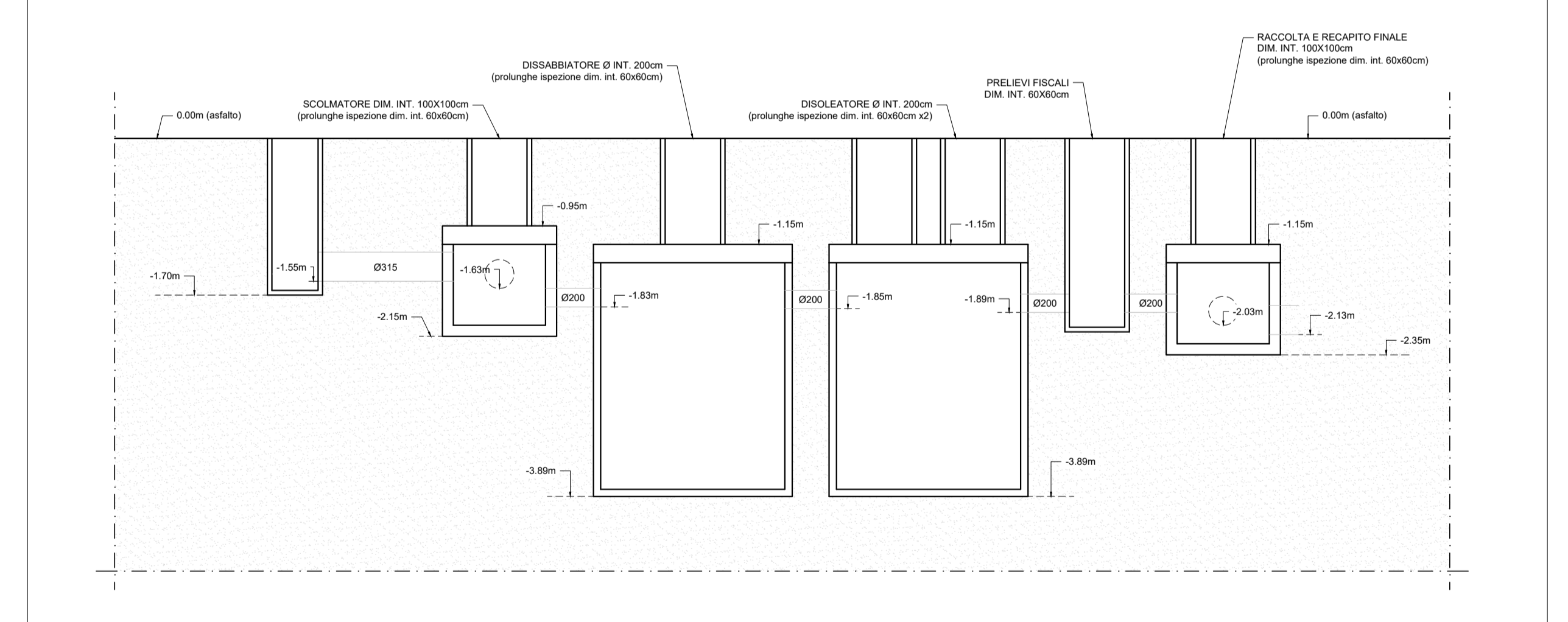
SEZIONE IMPIANTO PRIMA PIOGGIA (scala 1:50)
