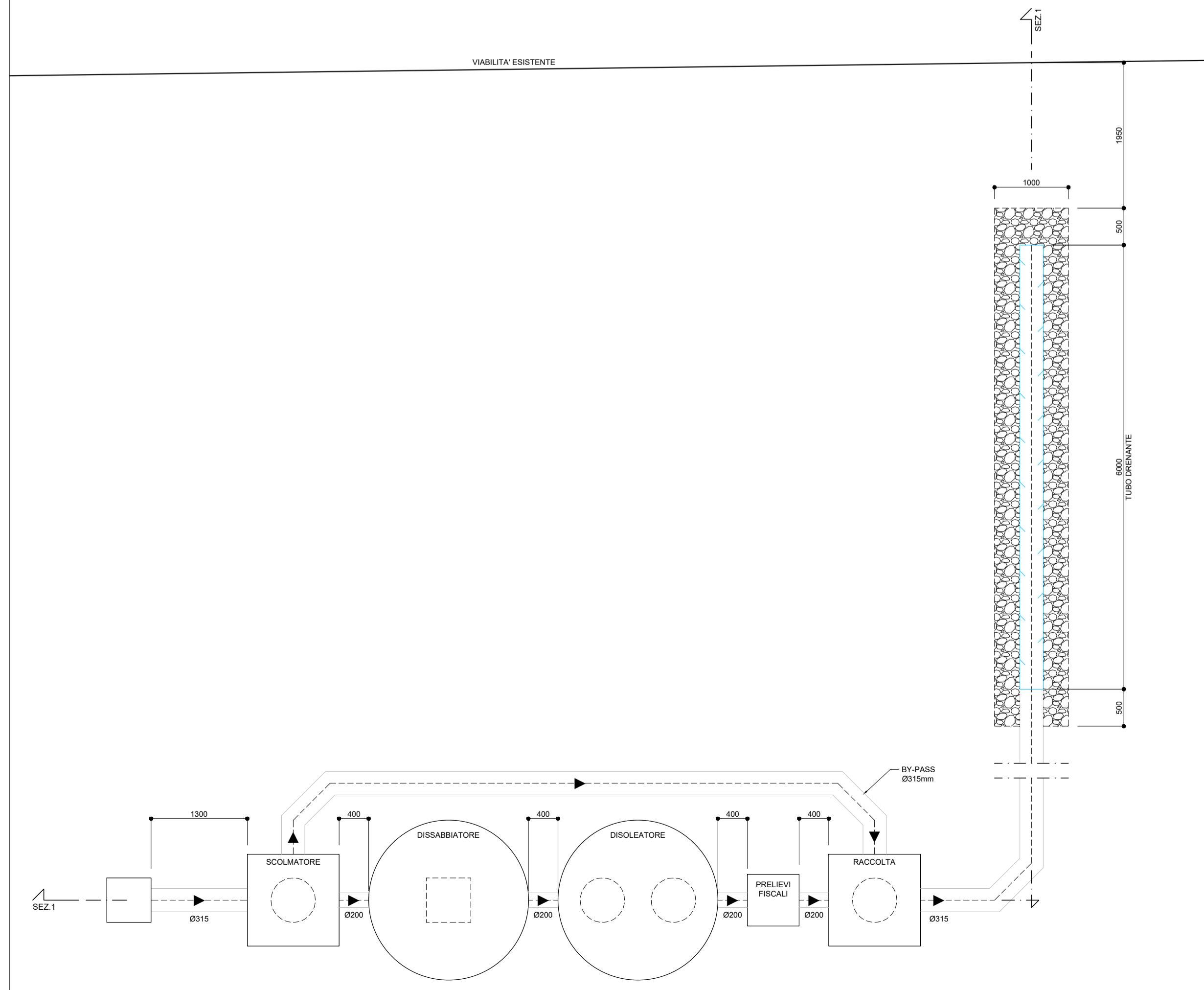
PIANTA IMPIANTO PRIMA PIOGGIA (scala 1:50)
