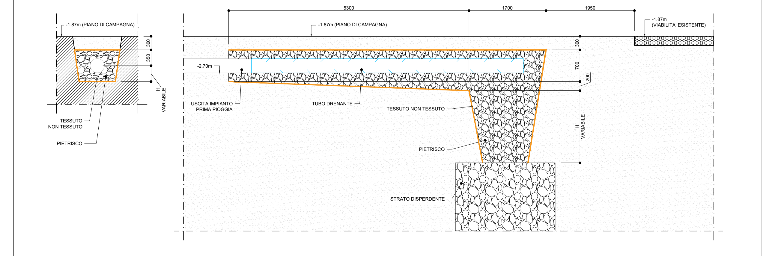
SEZIONI MATERASSO DRENANTE (scala 1:50)
