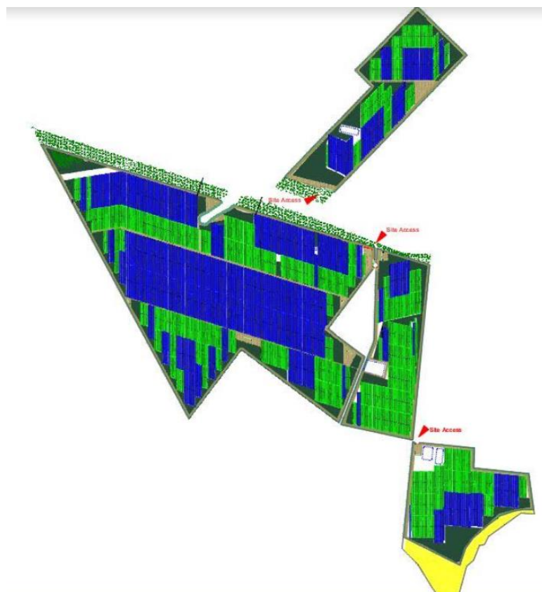
Layout dell'impianto fotovoltaico.
