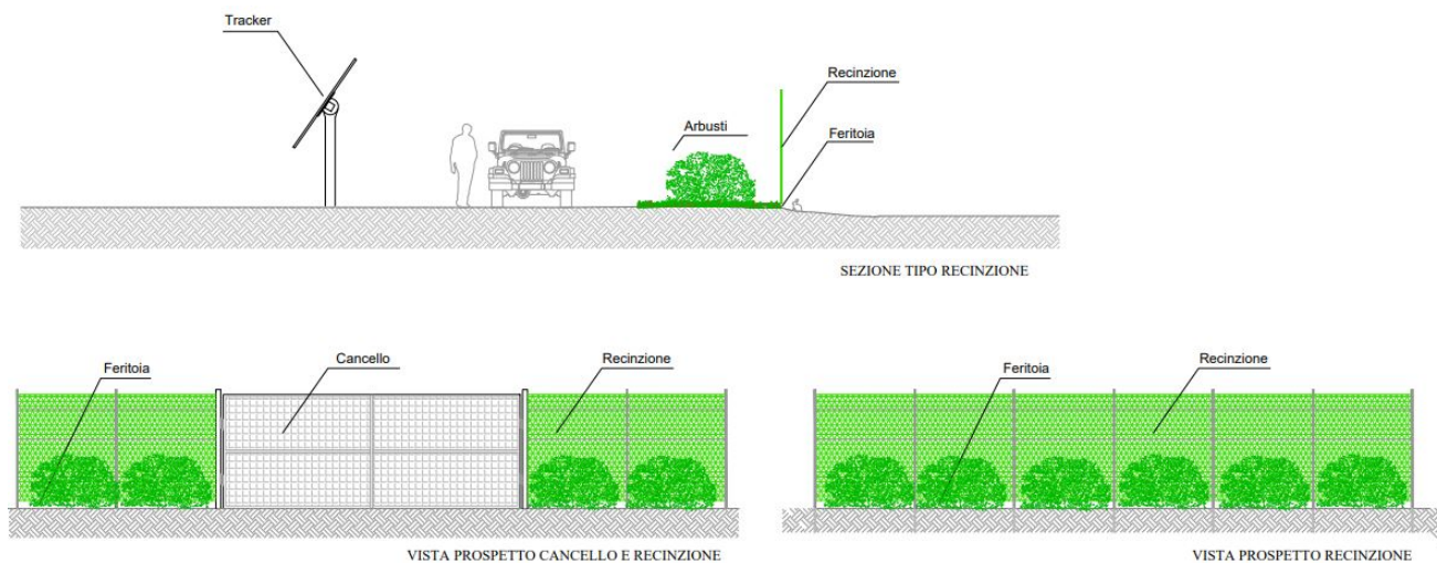
Figura 46 - Particolare della recinzione
