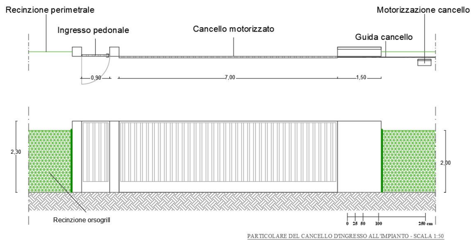
Figura 45 - particolare cancello di ingresso
