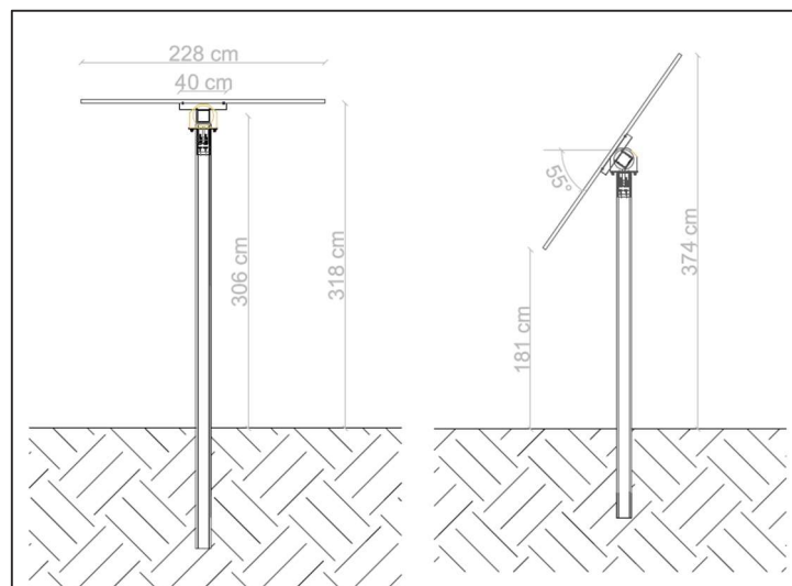
FIGURA 2: SCHEMA TIPO TRACKER AD ASSE VARIABILE
