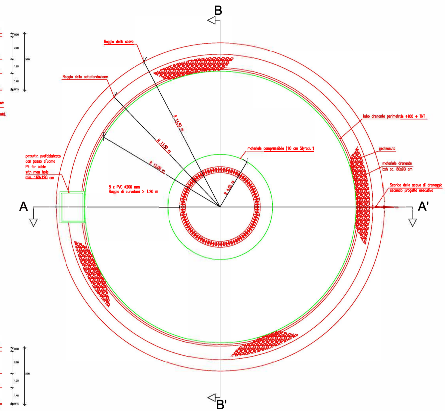
PIANTA
