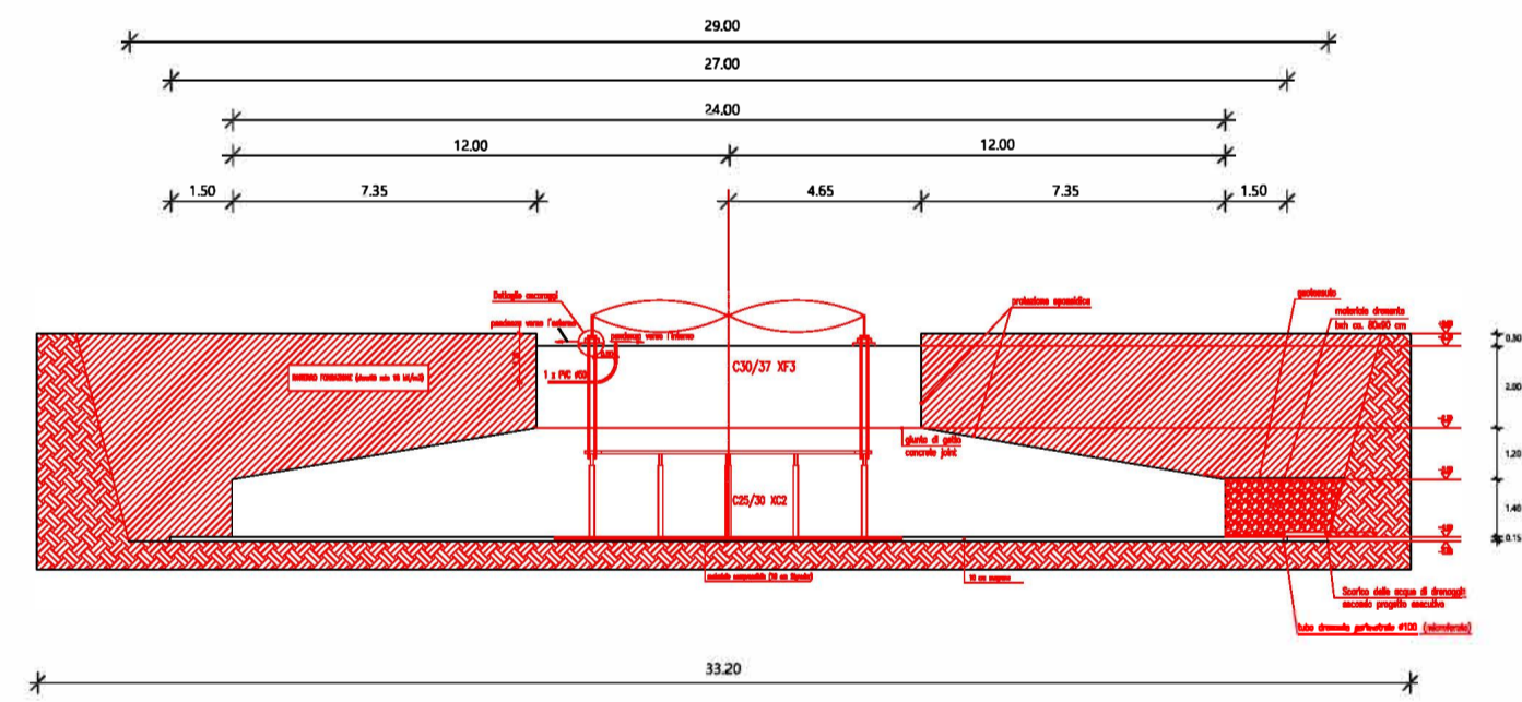
SEZIONE B-B'
