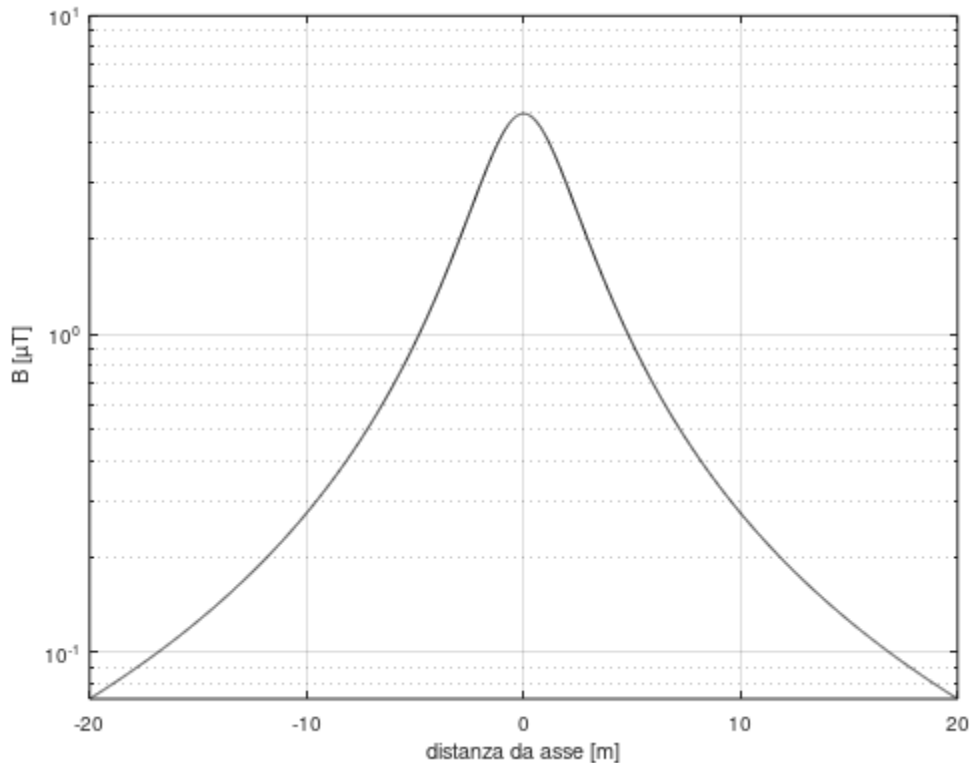
Figura 1: campo di induzione magnetica generato dalla linea in cavo interrato, percorsa dalla sua corrente nominale (725 A), con riferimento ad un'altezza di calcolo pari ad 1 m.
