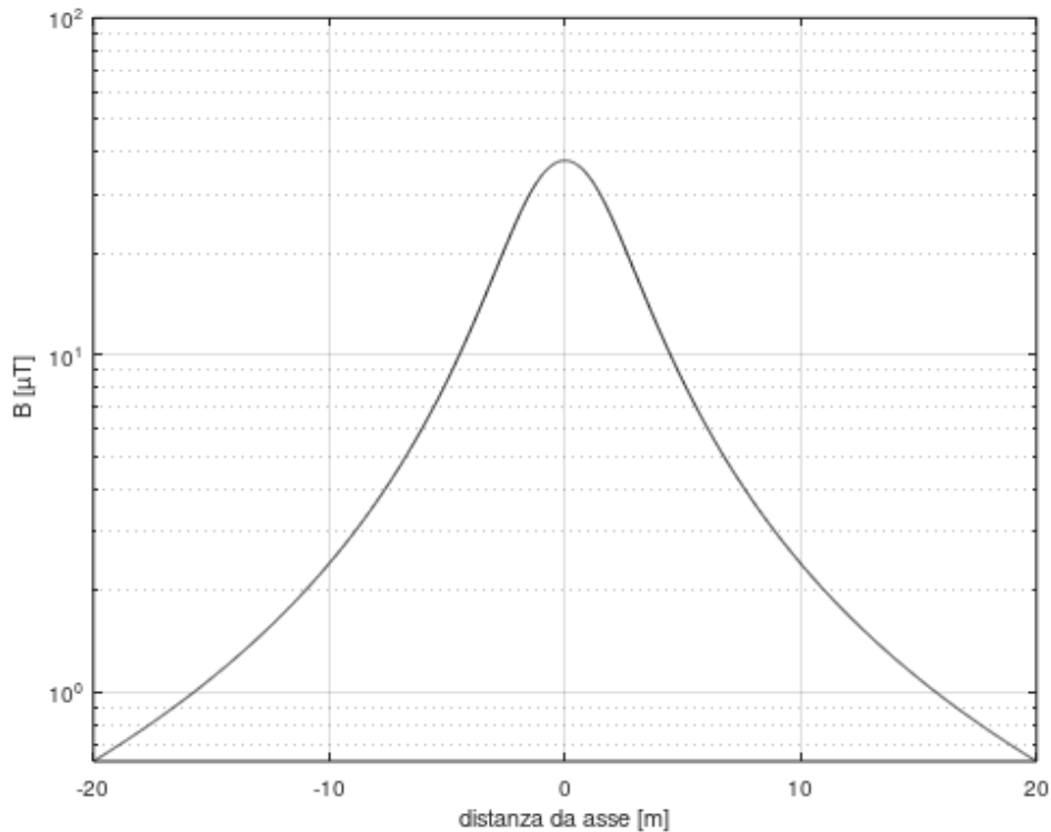
Figura 2: campo di induzione magnetica generato da una buca giunti della linea in cavo interrato, percorsa dalla sua corrente nominale (725 A), con riferimento ad un'altezza di calcolo pari ad 1 m.
