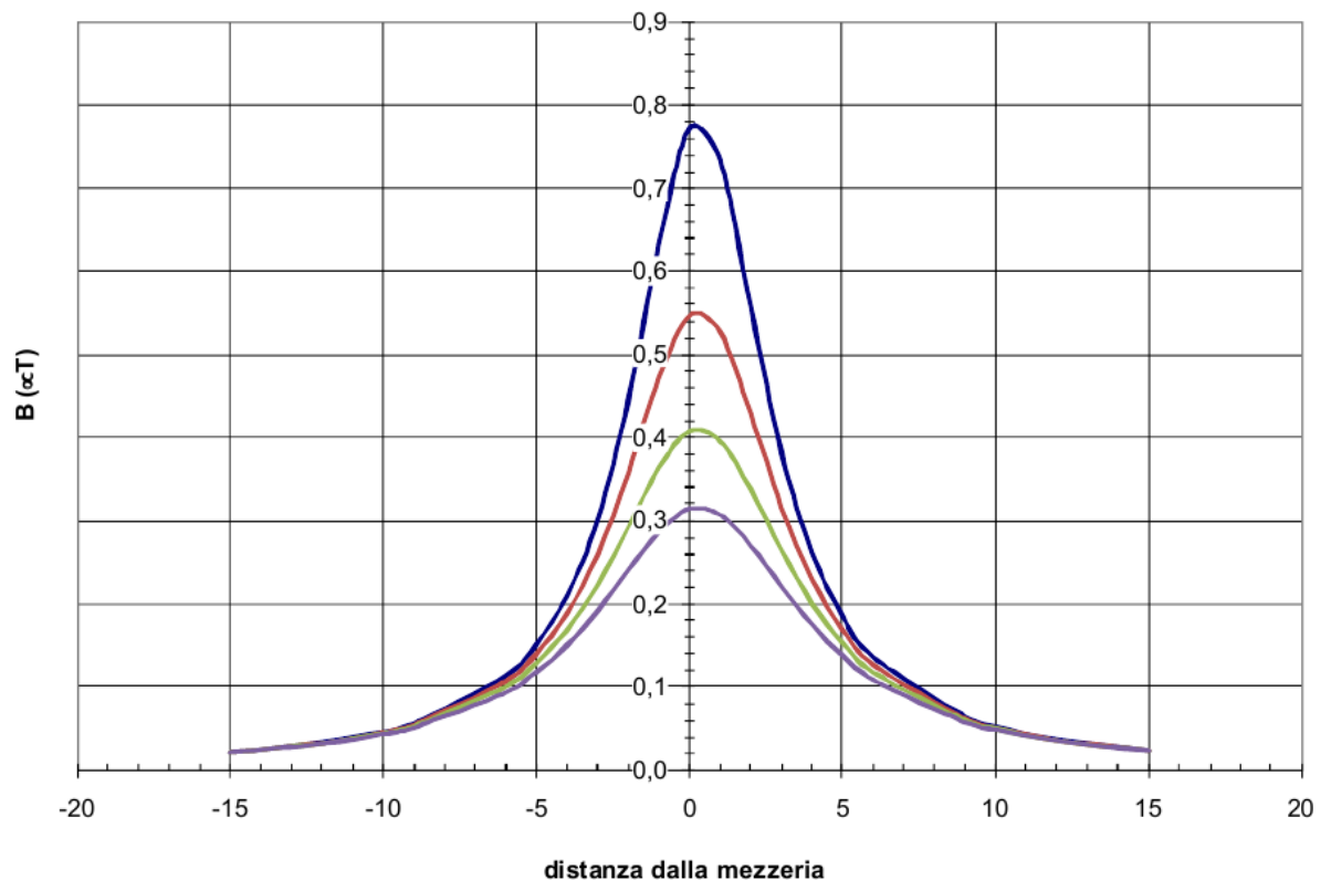
Figura 2. Andamento del campo magnetico in funzione della distanza di interrimento (Blu= 0.5m, rosso=1.0 m,verde=1.5m, viola =2m)
