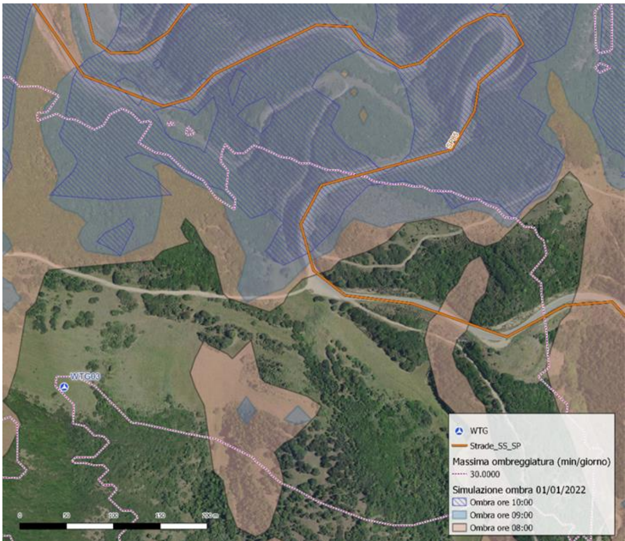
Figura 9: Simulazione ombreggiatura per strada SP85. In viola il perimetro della superficie che subisce ombreggiatura max giornaliera > 30 min/giorno a causa delle turbine del parco in proposta. Le superfici rosa, blu, tratteggiate corrispondono all'ombreggiatura dovuta al territorio (DTM, non DSM) limitrofo alle ore 08,09,10AM rispettivamente. Sono ottenute via simulazione r.sunmask.position (GRASS) impostata al 01/01/2022 e non sono dovute a nessuna WTG, ma solo al territorio circostante.
