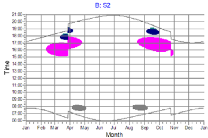
Figura 10: calendario grafico ombreggiatura delle WTG sulla SP85 nell'area dove l'ombra massima giornaliera > 30min/giorno (fig.9). In grigio WTG04, in fuxia WTG03 e in blu WTG02. Questa immagine è ricavata dallo scenario "caso peggiore", senza tenere conto di eliofania e rosa dei venti.
