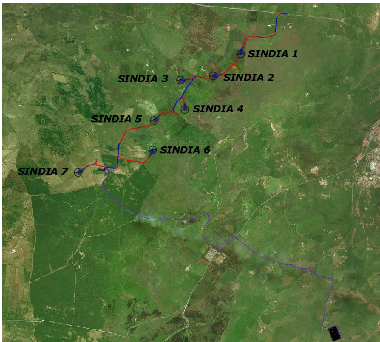
Figura 1 Localizzazione su base satellitare su base ortofoto degli aerogeneratori
