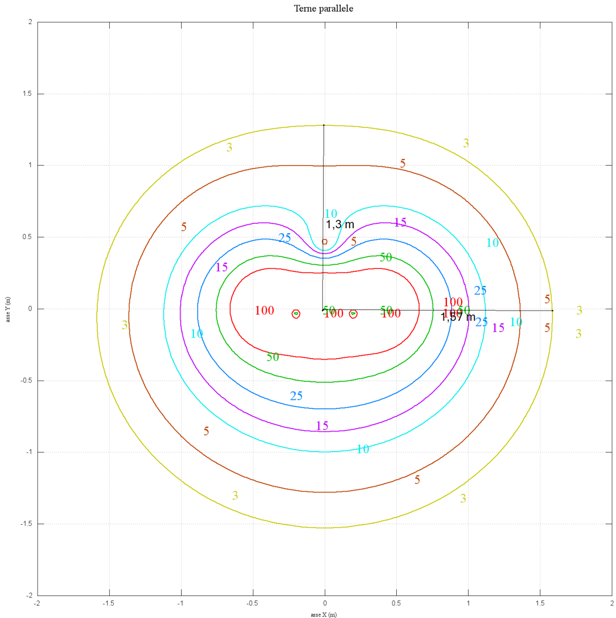
Figura 10 - Curve di isolivello AT
