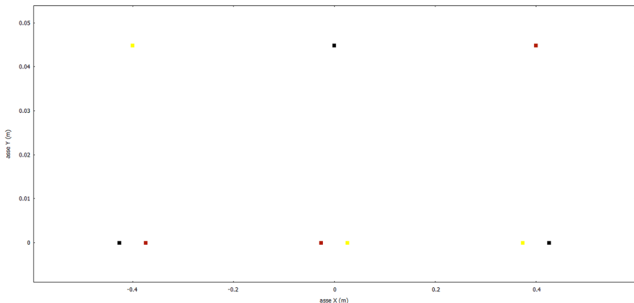
Figura 9 – Geometria disposizione cavi AT.
