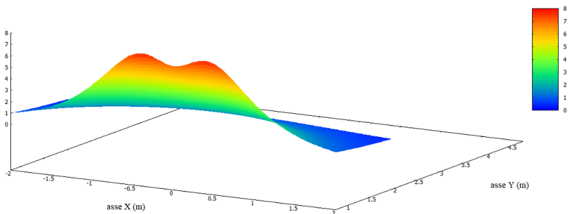
Figura 3 - Ulteriore simulazione cavidotto AT con tre terne a 36kV.
