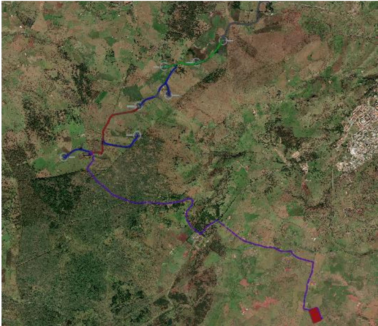
Figura 1: Inquadramento su base IGM – in magenta il cavidotto a 36 kV
