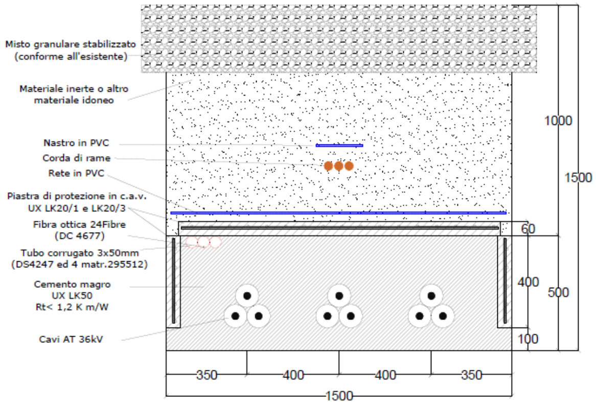
Figura 2 - Sezione cavidotto AT con tre terne su strada sterrata (Sezione C-C')
