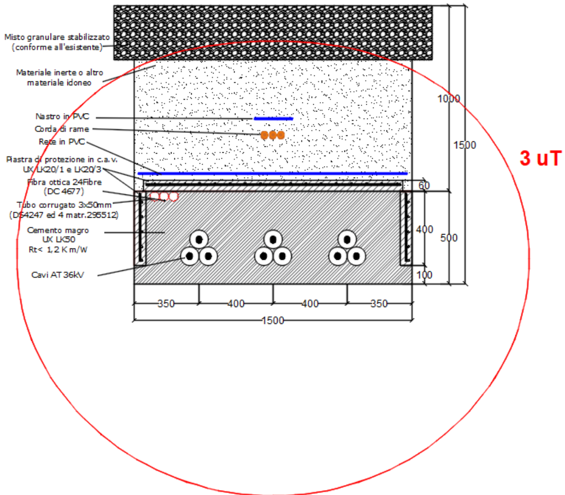
Figura 11 - Curva isolivello su sezione AT
