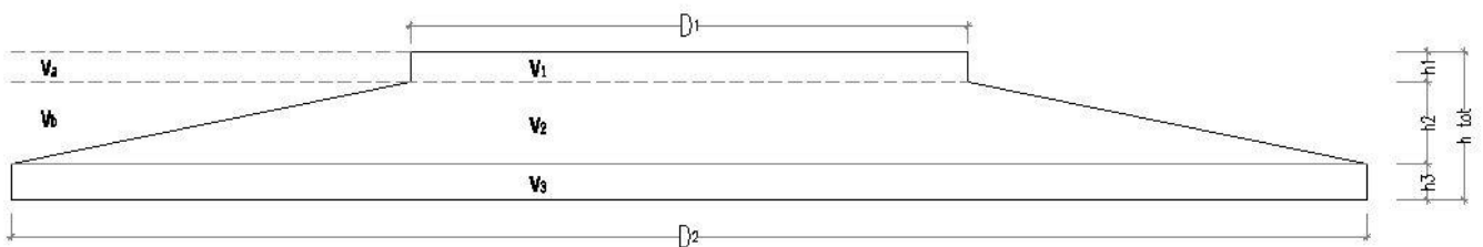
Schema in sezione basamento di fondazione
