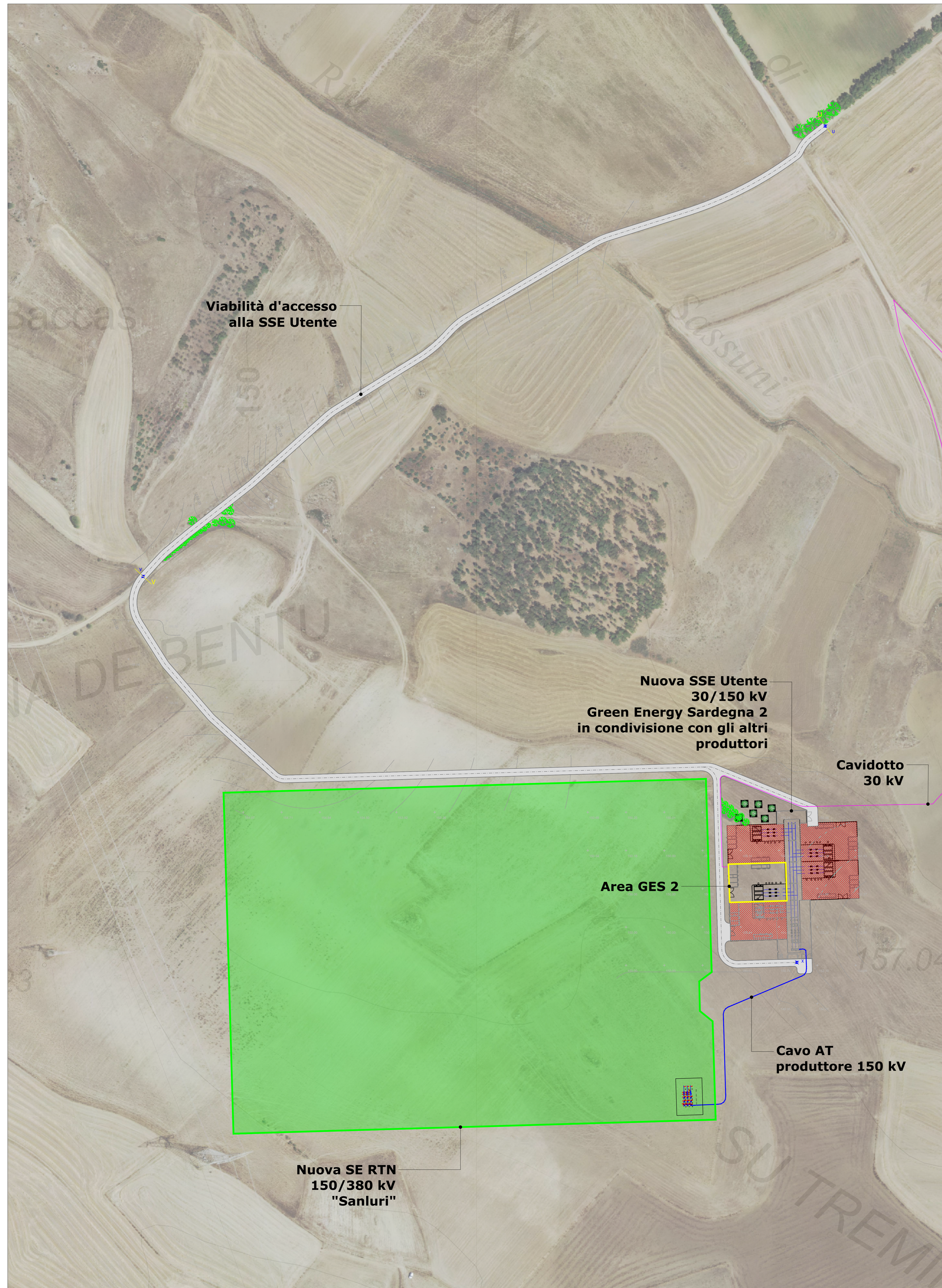
INQUADRAMENTO SU ORTOFOTO - STATO DI PROGETTO - SC.1:1.000
