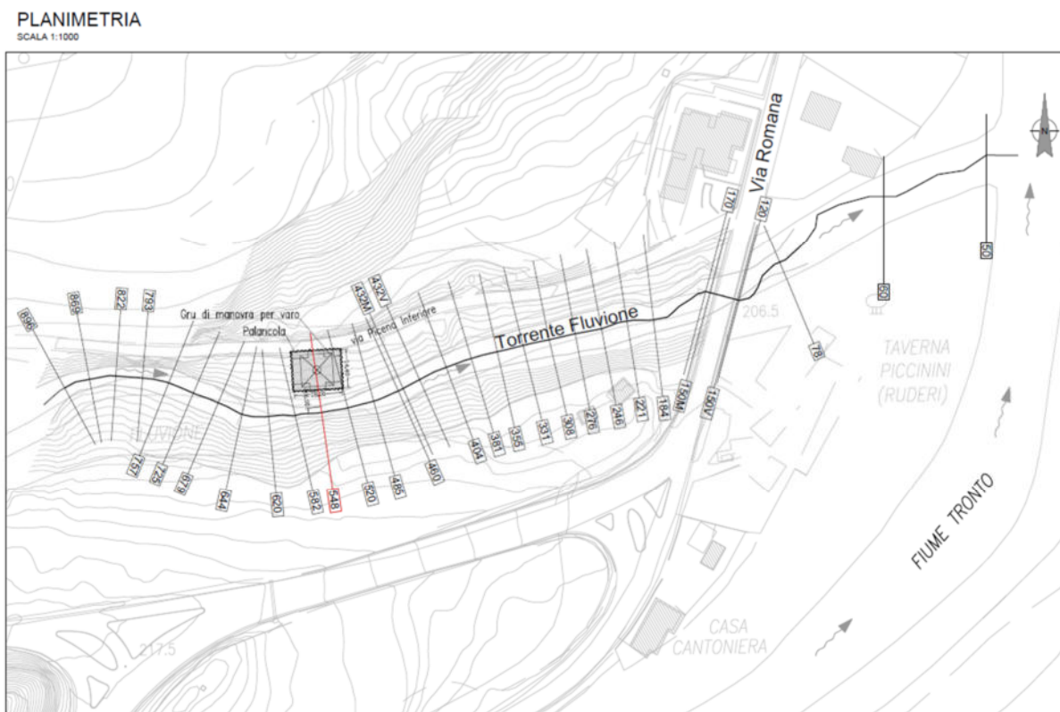
Figura 3-1 – Planimetria con indicazione delle sezioni trasversali utilizzate nella modellazione
