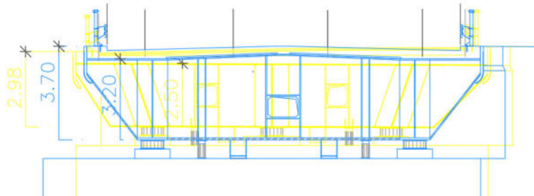
Figura 4-2 – Sezione in asse appoggi Spalla PD-PE
