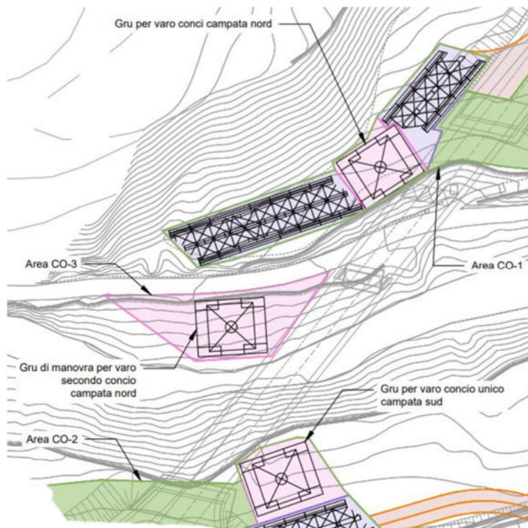
Figura 4-6 – Presenza della Gru per il Varo dal basso – Progetto definitivo
