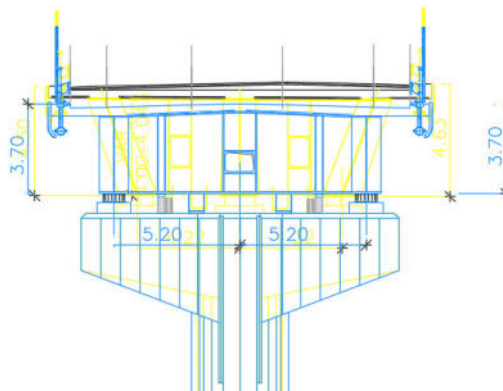
Figura 4-3 – Sezione in asse Pila PD-PE
