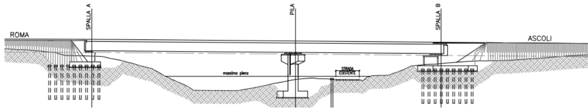
Figura 3-2 – Schema delle fasi costruttive del Viadotto Fluvione con modalità di varo a spinta in fase di progettazione esecutiva
