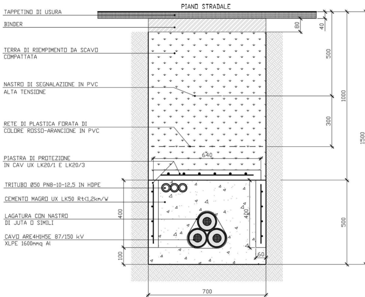
Fig. 21 – Sezione di posa a trifoglio sotto strada
