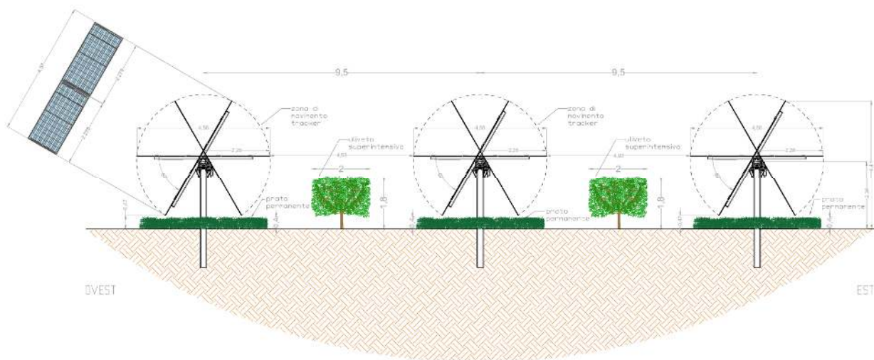
Fig. 1 Sistema Agrivoltaico
