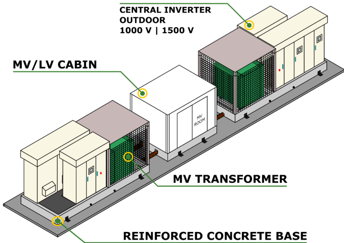
Fig. n°16 Power Skid
