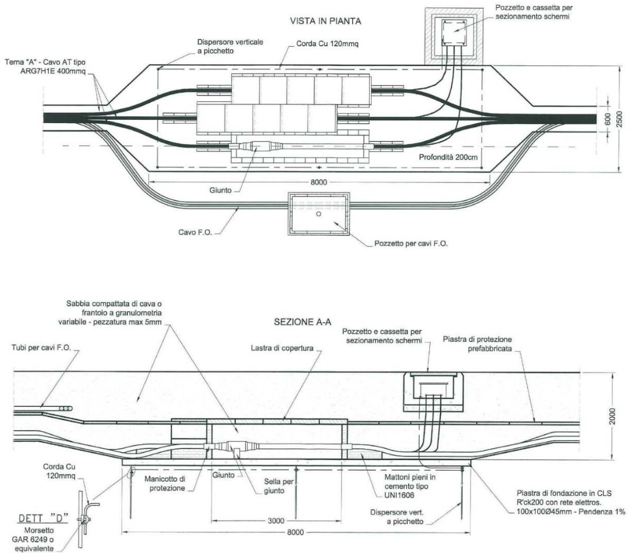
Fig.23 – Tipica buca giunti
