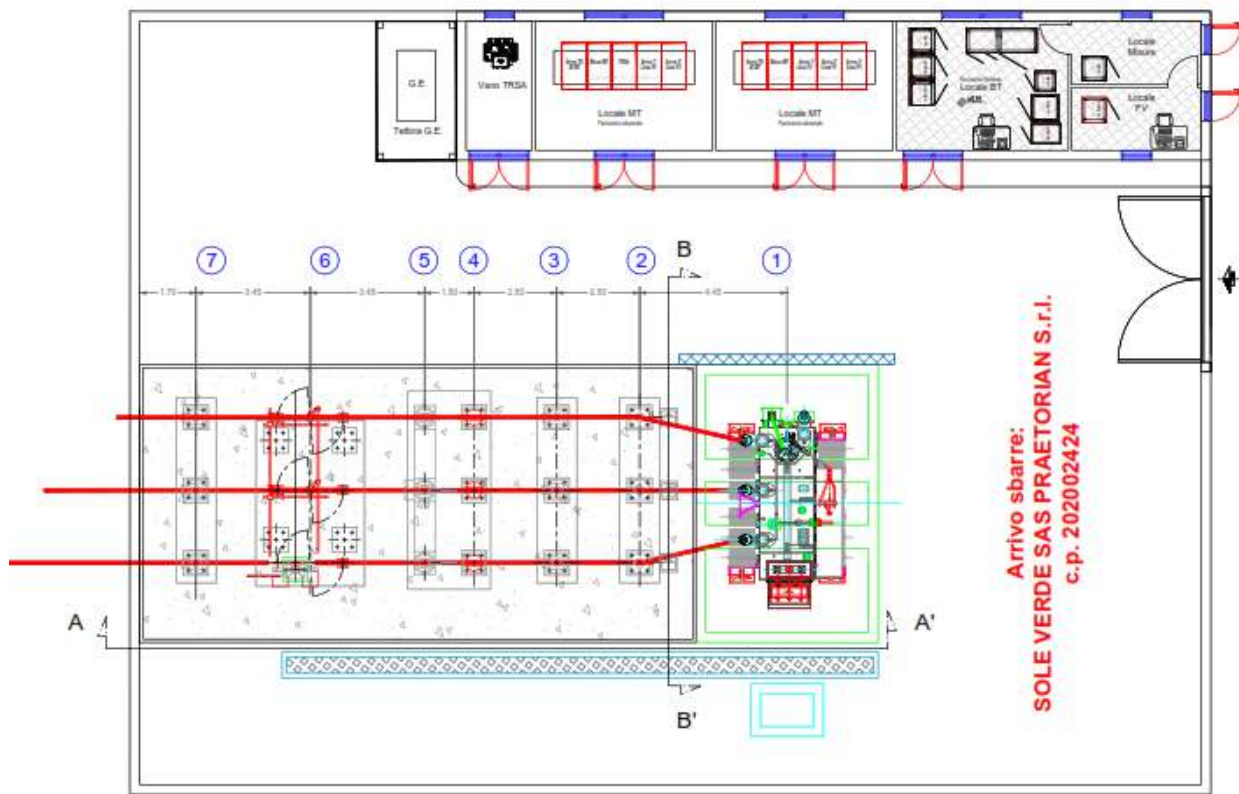
Fig. 12 Planimetria sottostazione utente
