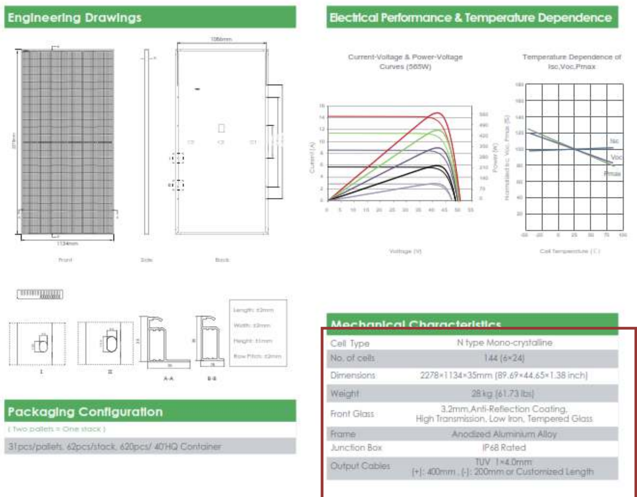
Fig. 8 Data Sheet Modulo Fotovoltaico _1
