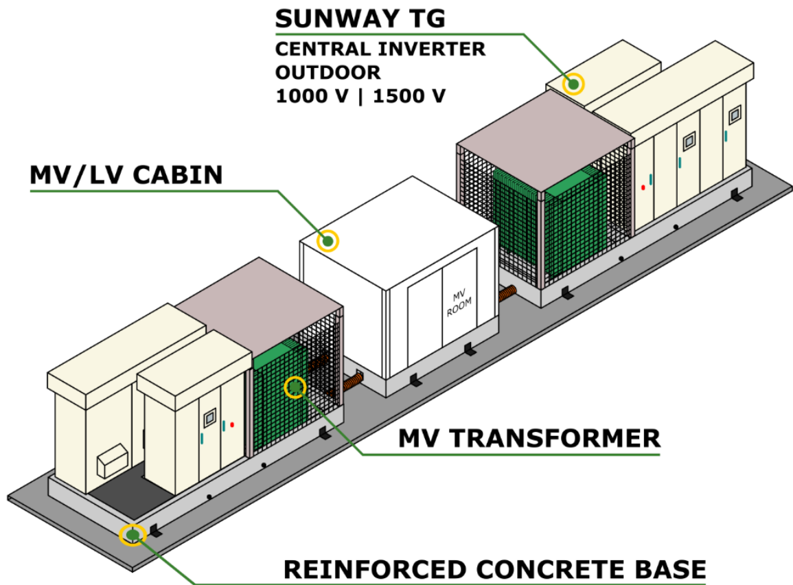
Fig. n°11 Power Skid
