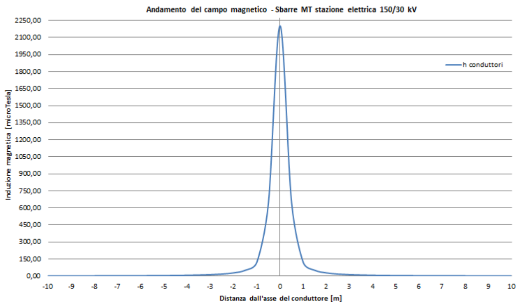
Figura 6 Andamento del campo magnetico in funzione della distanza dall'asse dei conduttori in forma grafica - Sbarre MT stallo di trasformazione di progetto 30/150 kV - Valutazione della Distanza di prima Approssimazione.
