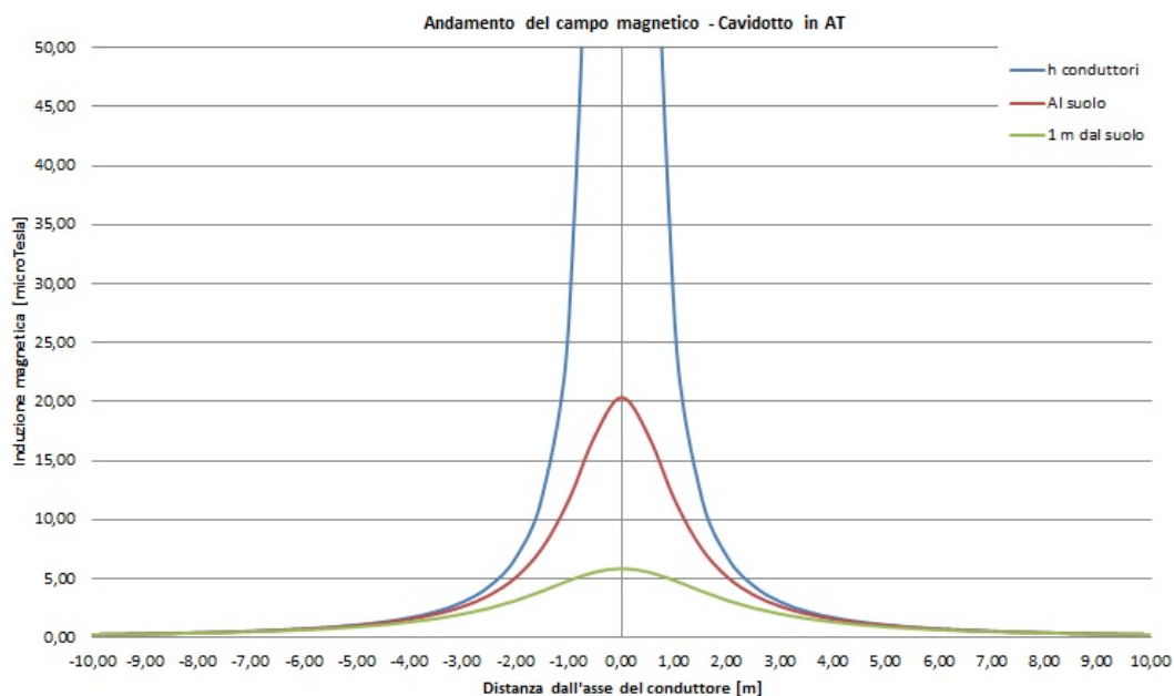
Figura 10 Rappresentazione grafica della DPA cavidotto AT 150 kV.
