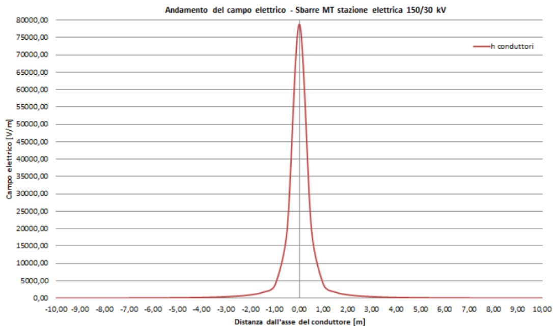
Figura 8 Andamento del campo elettrico in forma grafica – Sbarre MT stallo di trasformazione di progetto 30/150 kV.
