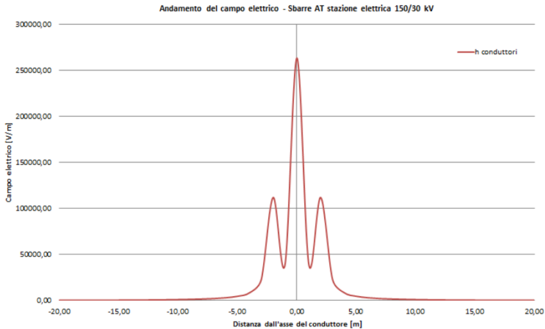
Figura 7 Andamento del campo elettrico in forma grafica - Sbarre AT stallo di trasformazione di progetto 30/150 kV.
