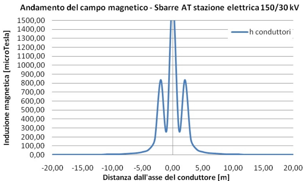
Figura 5 Andamento del campo magnetico in funzione della distanza dall'asse dei conduttori in forma grafica - Sbarre AT stallo di trasformazione di progetto 30/150 kV - Valutazione della Distanza di prima Approssimazione.
