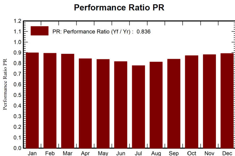
Figura 3: Indice di rendimento (Performance Ratio)
