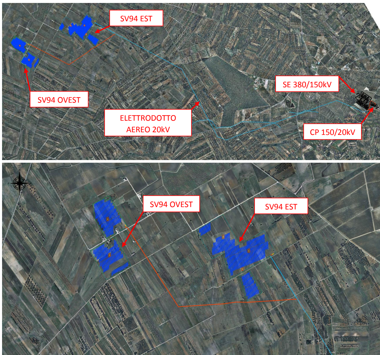
Figura 4: Layout di progetto
