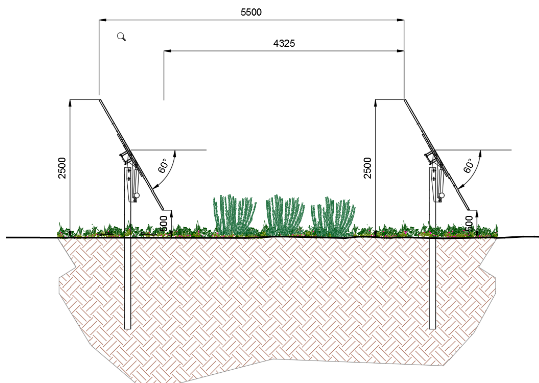
Figura 5: sezioni trasversale delle strutture di sostegno
