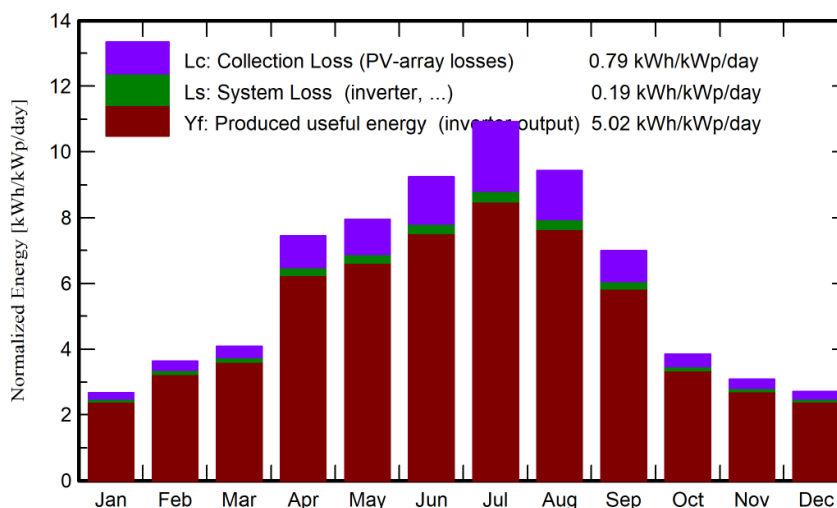
Figura 2: Istogramma energia normalizzata prodotta e perdite durante anno solare per kWp installato
