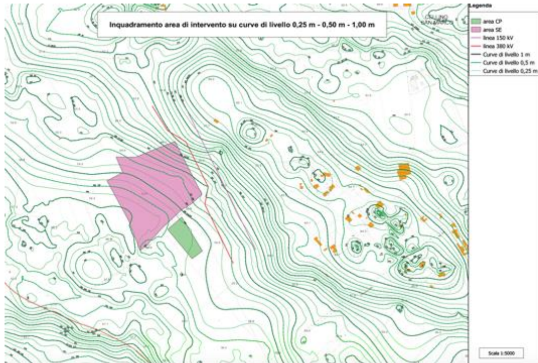
Tavola n. 10: Rilievo topografico con isoipse dell'ordine di 0,25 m., 0,50 m. e 1 m.
