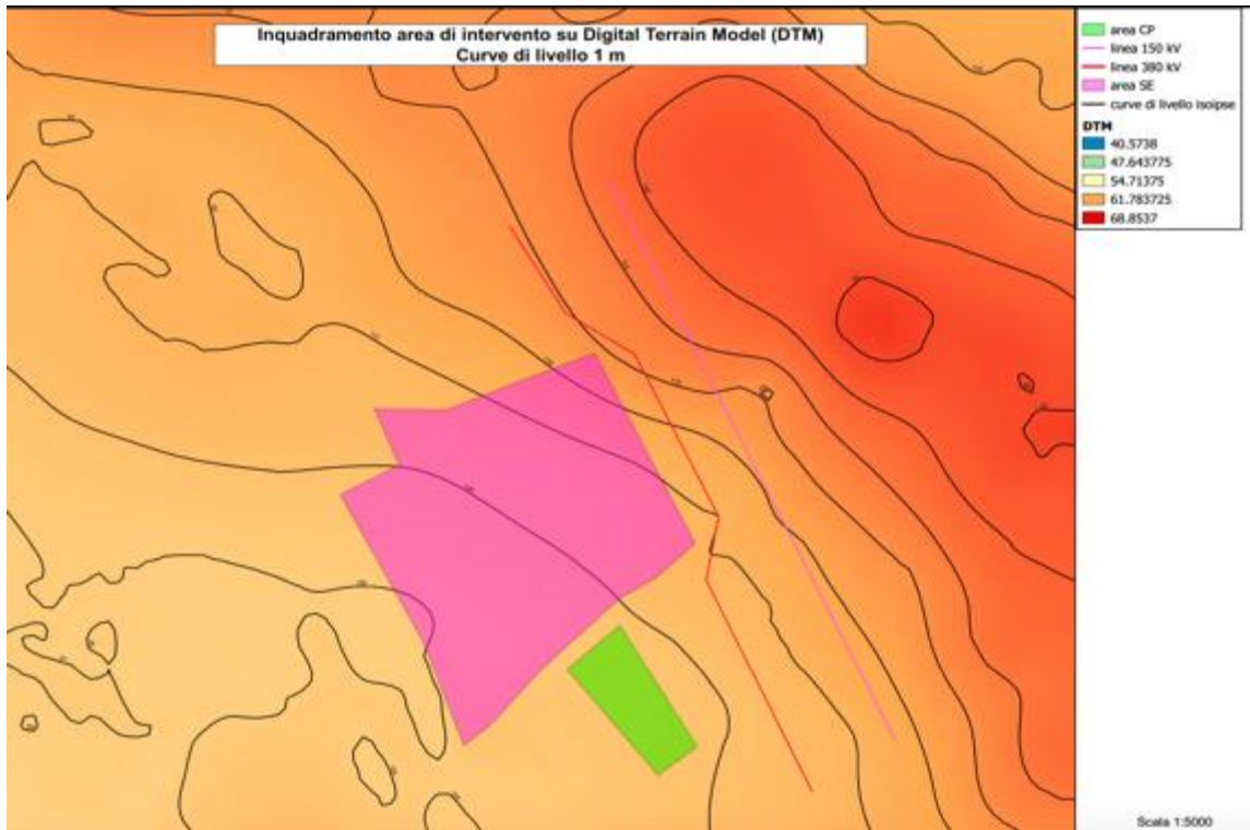
Tavola n. 11: Inquadramento con "digital terrain model" (DTM)
