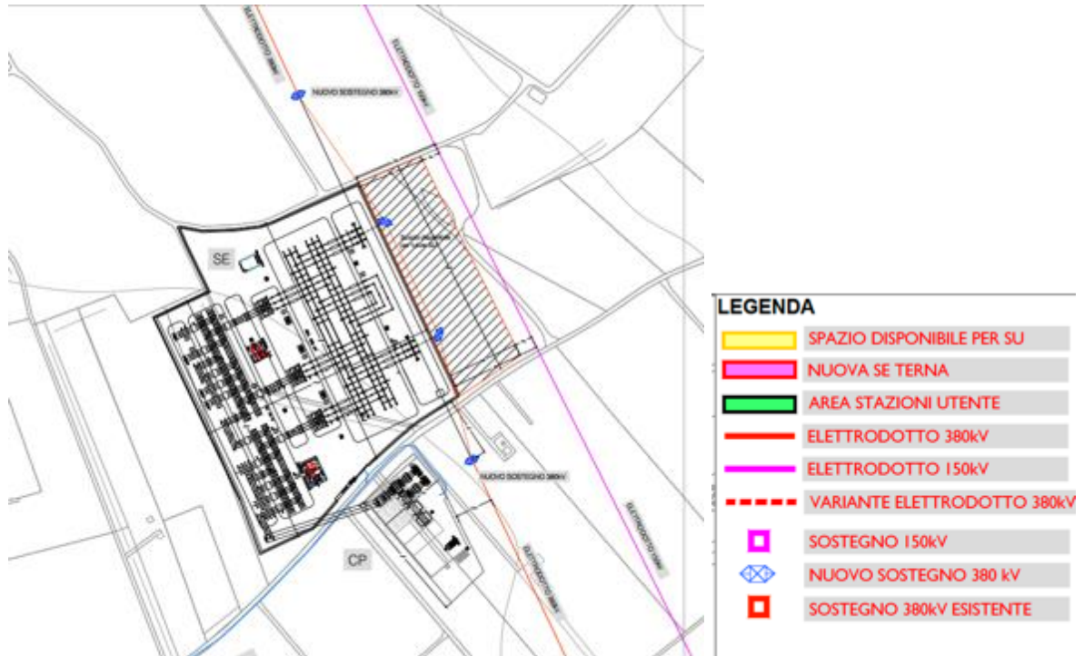
Tavola n. 5: Inquadramento catastale della SE e della CE.
