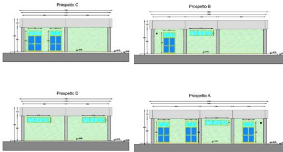
Figura 3: Prospetti edificio Servizi Ausiliari
