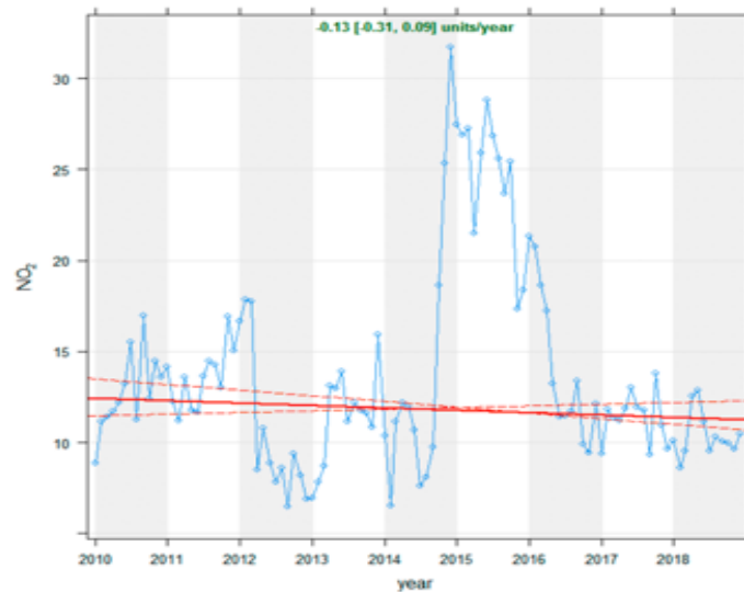
Tavola n. 11: NO2 -Andamento delle medie annuali nell'arco temporale 2010-2018.
