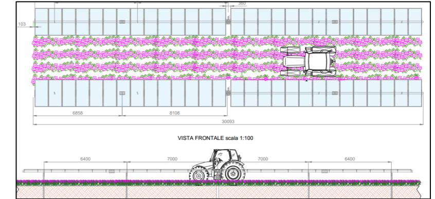
Tipici strutture porta moduli e schema culturale
