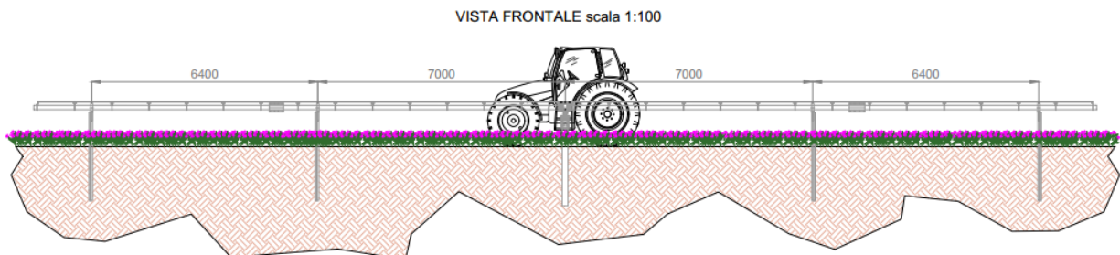
Fig. 3 - Schema della struttura – vista longitudinale
