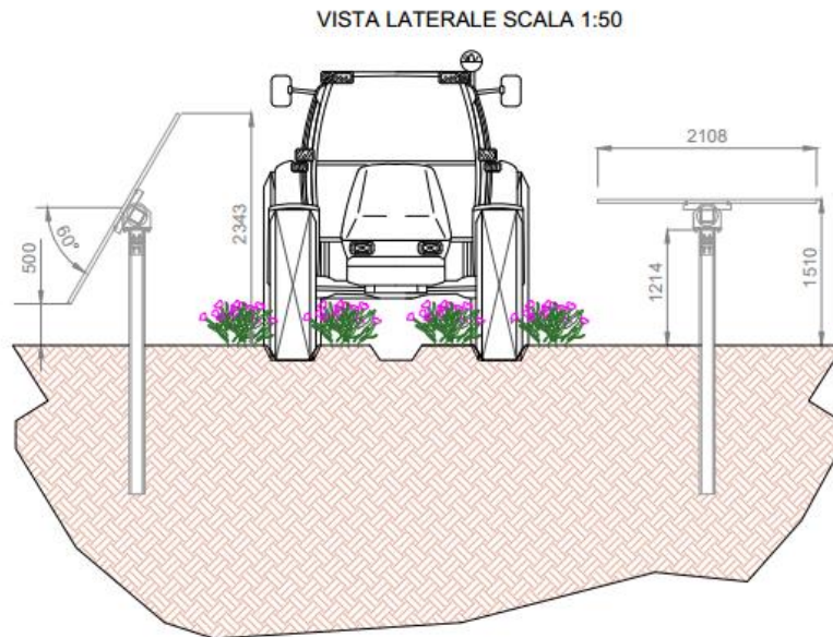
Fig. 2 - Schema della struttura – sezione
