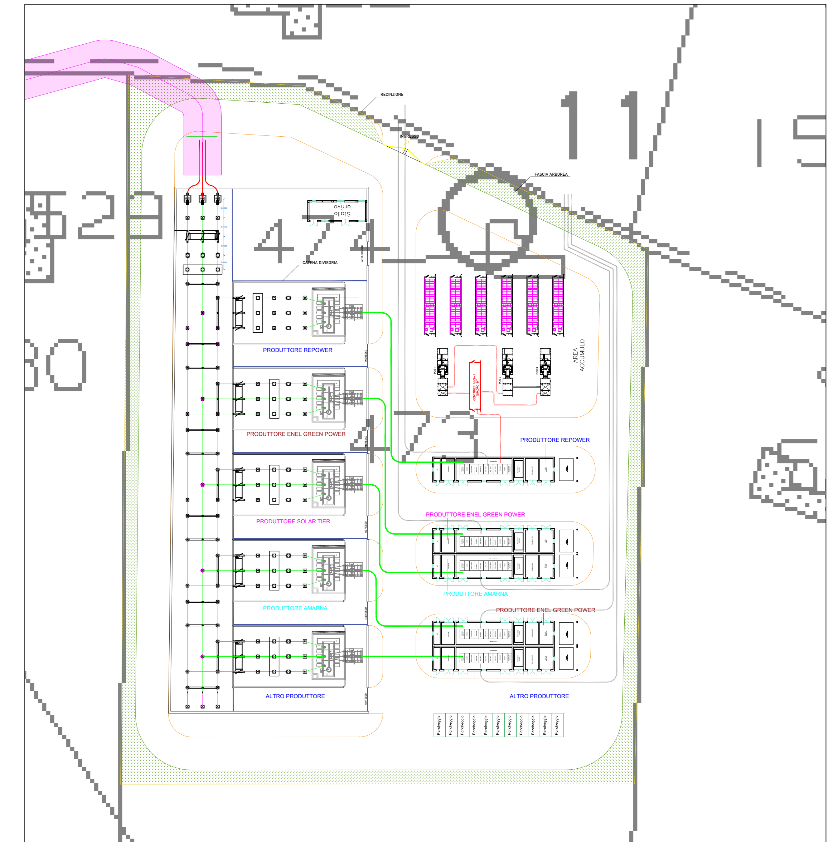
INQUADRAMENTO SU CATASTALE (fg.52 comune di SANTA NINFA) SSE REPOWER_STALLO SOLAR TIER scala 1:500
