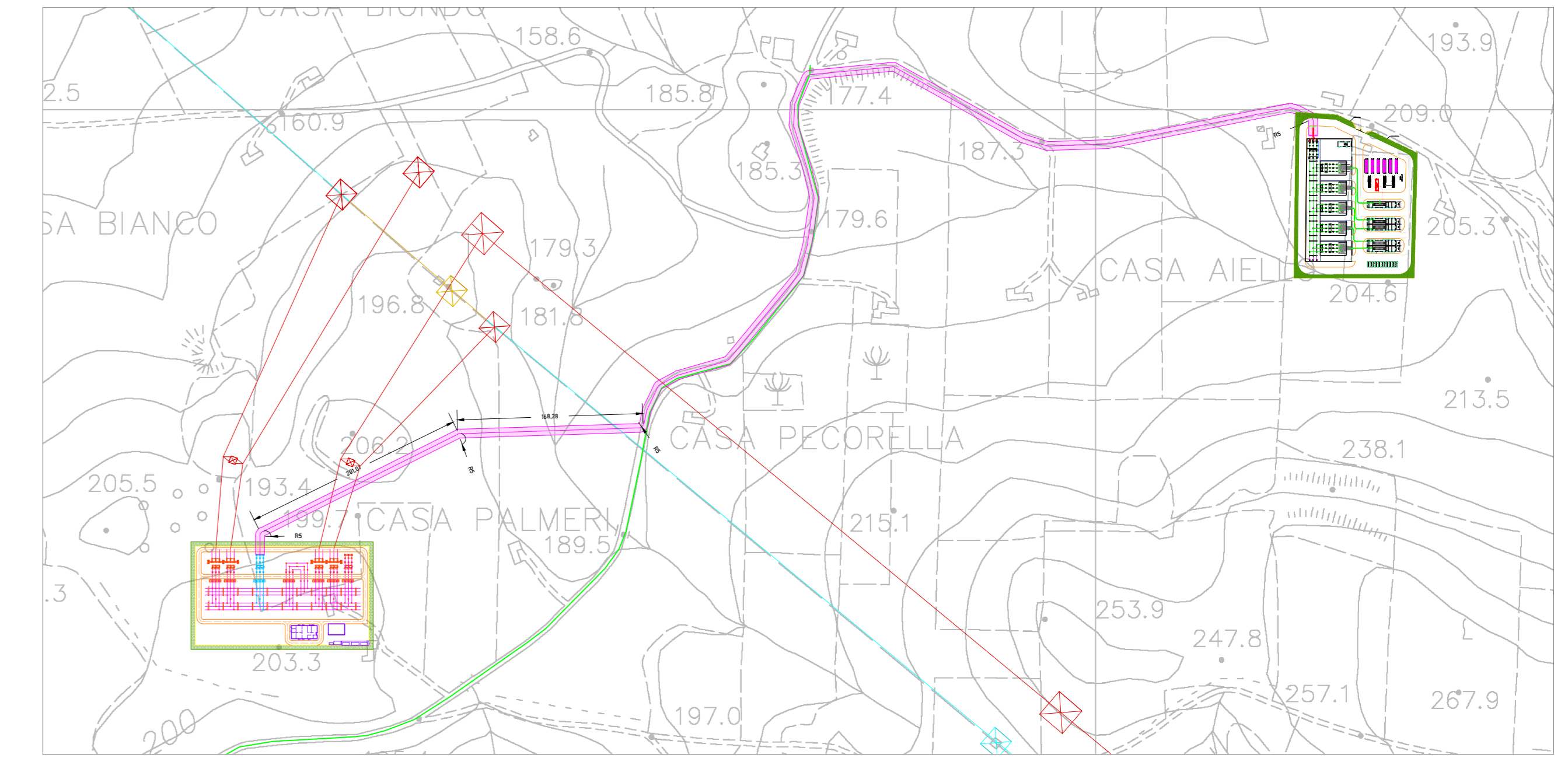
INQUADRAMENTO SU CTR - scala 1:4.000
