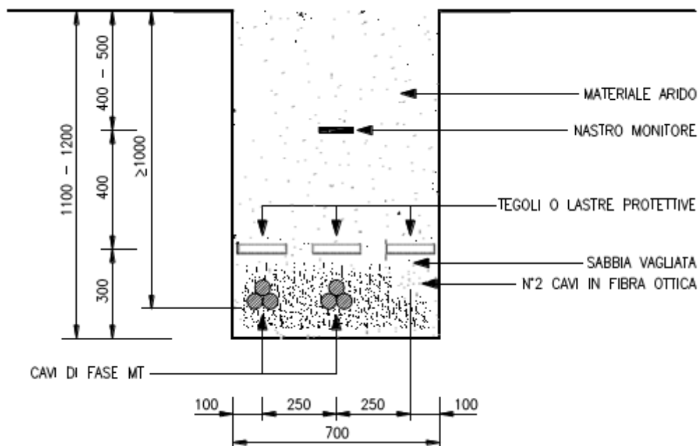
Figura 4 - Sezione tipica di posa della linea di cavo
