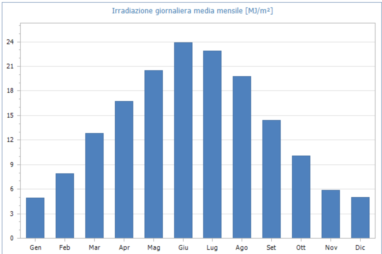
Fig. 1: Irradiazione giornaliera media mensile sul piano orizzontale [MJ/m²]- Fonte dati: UNI 10349:2016 - Stazione di rilevazione: Sassari
