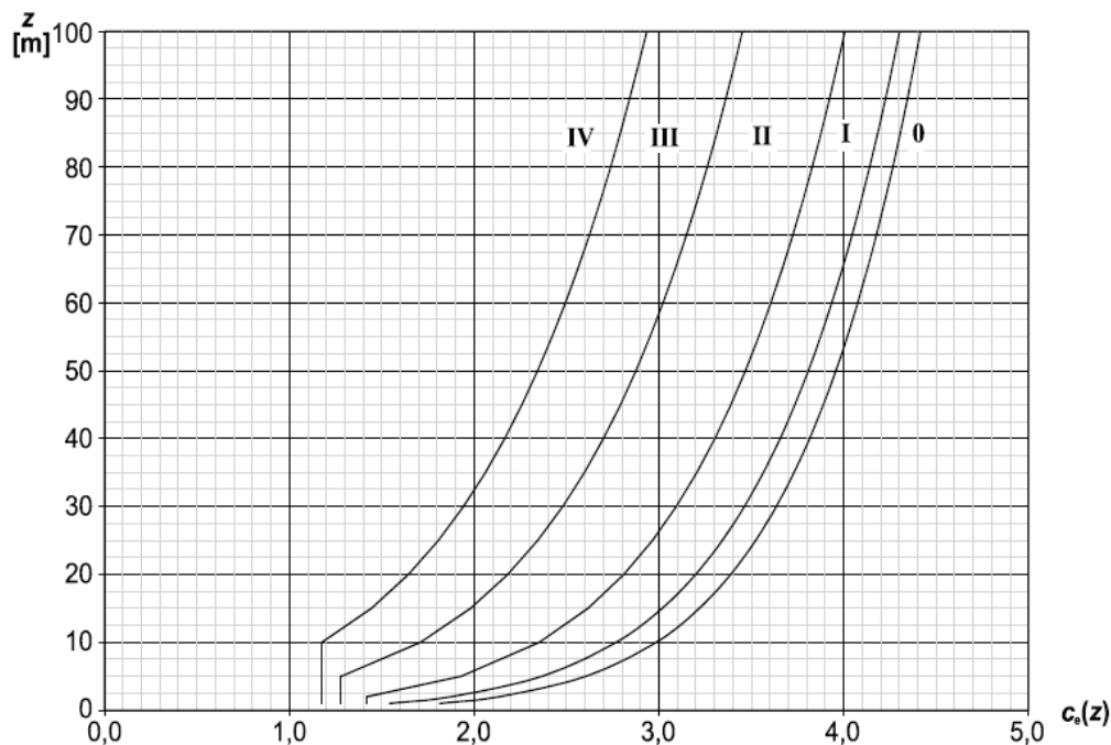
Figura 1 – Andamento del coefficiente d'esposizione C_e(z) con la quota (per c_t = 1 )
