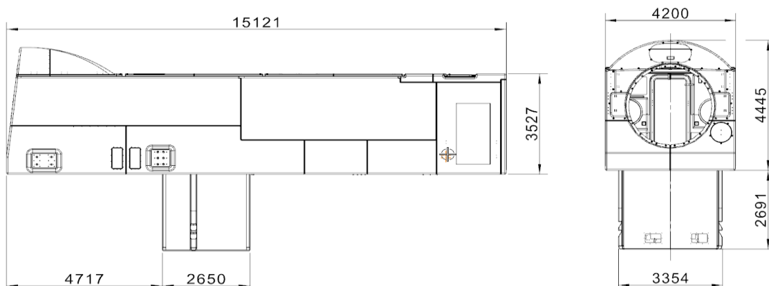
Figura 1- Schema aerogeneratore
