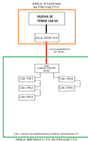
FIGURA 5: SCHEMA A BLOCCHI IMPIANTO
