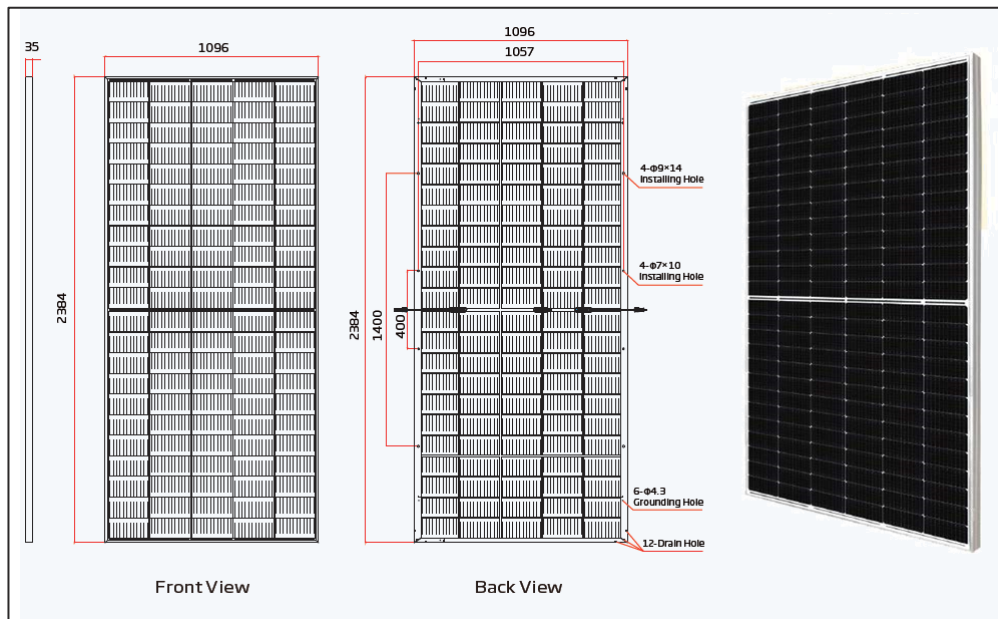
FIGURA 6: PANNELLO FV PARI A 550 Wp CON DIMENSIONI 2384 X 1096 X 35 MM
