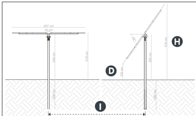
FIGURA 3: DEFINIZIONE DELLE DIMENSIONI DEI TRACKER
