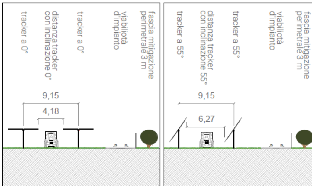
FIGURA 38 – SEZIONI RAPPRESENTATIVE IMPIANTO CON MODULI IN POSIZIONE DI MANUTENZIONE A 0° (A SINISTRA) E 55° (A DESTRA) - ESTRATTO DALL'ELABORATO GRAFICO SASSARI3-PDT11)
