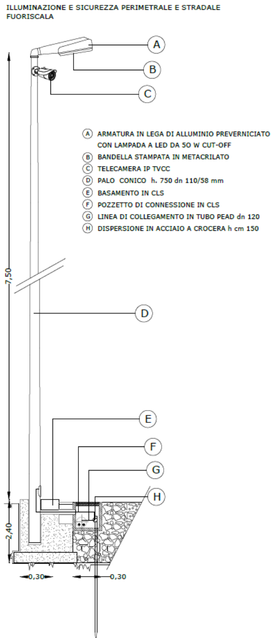
FIGURA 20 – ESEMPIO IMPIANTO DI ILLUMINAZIONE INTEGRATO CON SISTEMA DI VIDEOSORVEGLIANZA – ESTRATTO DALL'ELABORATO TECNICO SASSARI3-PDR02
