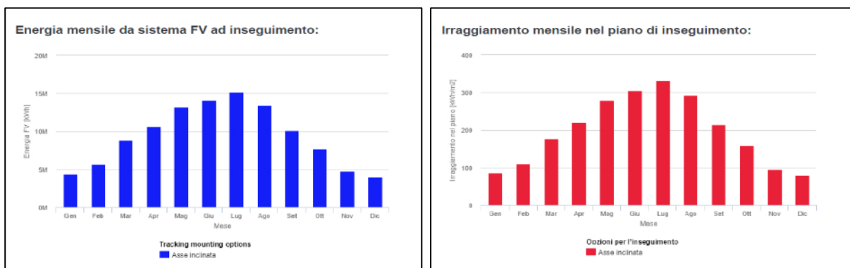
FIGURA 18 – SULLA SINISTRA PRODUCIBILITÀ MEDIA MENSILE DEL SITO, SULLA DESTRA IRRAGGIAMENTO AL METRO QUADRO – INFORMAZIONE ESTRATTA DALLA RELAZIONE TECNICA GENERALE PPTORESS-PDR01
