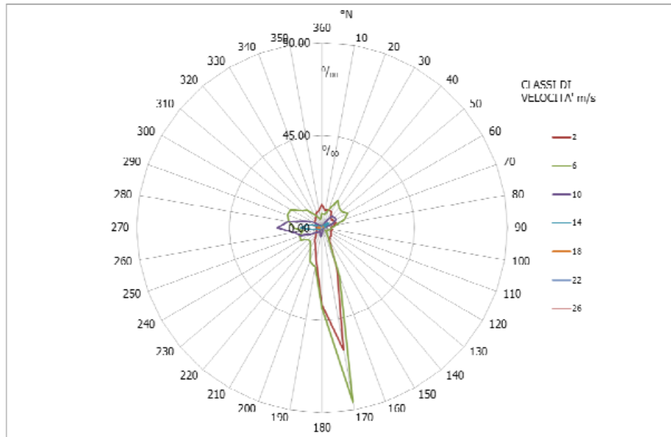
FIGURA 25 –ROSA DEL REGIME DEI VENTI NELLA STAZIONE DI PORTO TORRES CON DATI DI RILEVAMENTO DAL 23/07/98 AL 18/12/2010.
