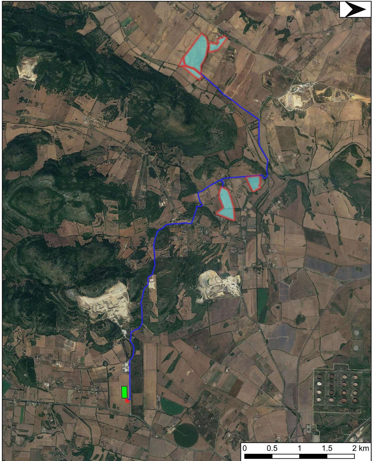
Figura 3.6-8 - Localizzazione impianto e cavidotto
