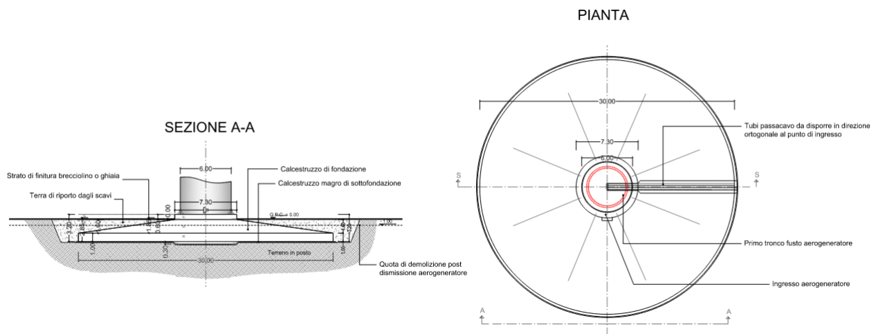
Figura 1 – Pianta e vista della fondazione tipo dell'aerogeneratore
