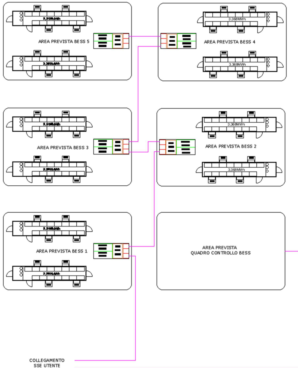
Figura 5 – Layout dell’impianto BESS all’interno dell’area disponibile
