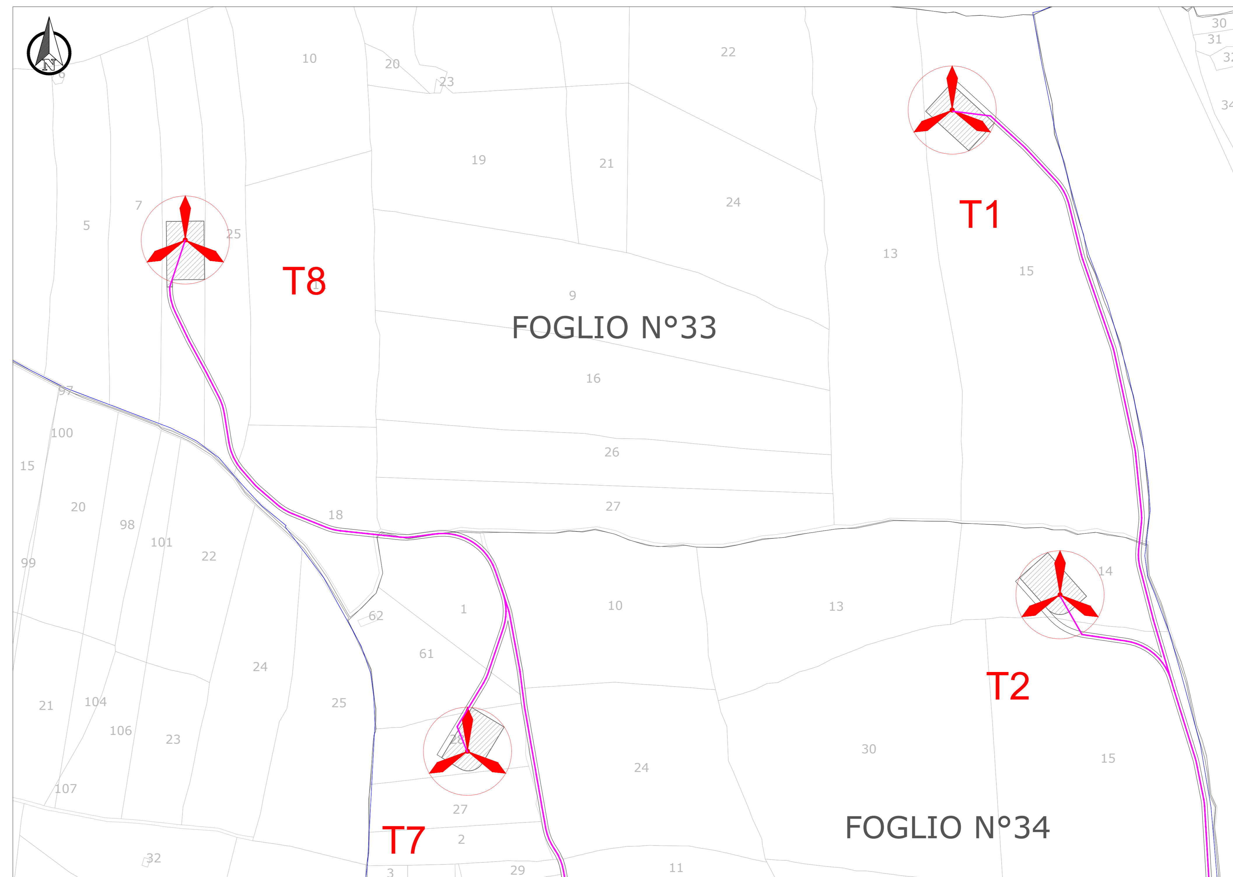
PLANIMETRIA CATASTALE - QUADRO C - Scala 1:2.000
