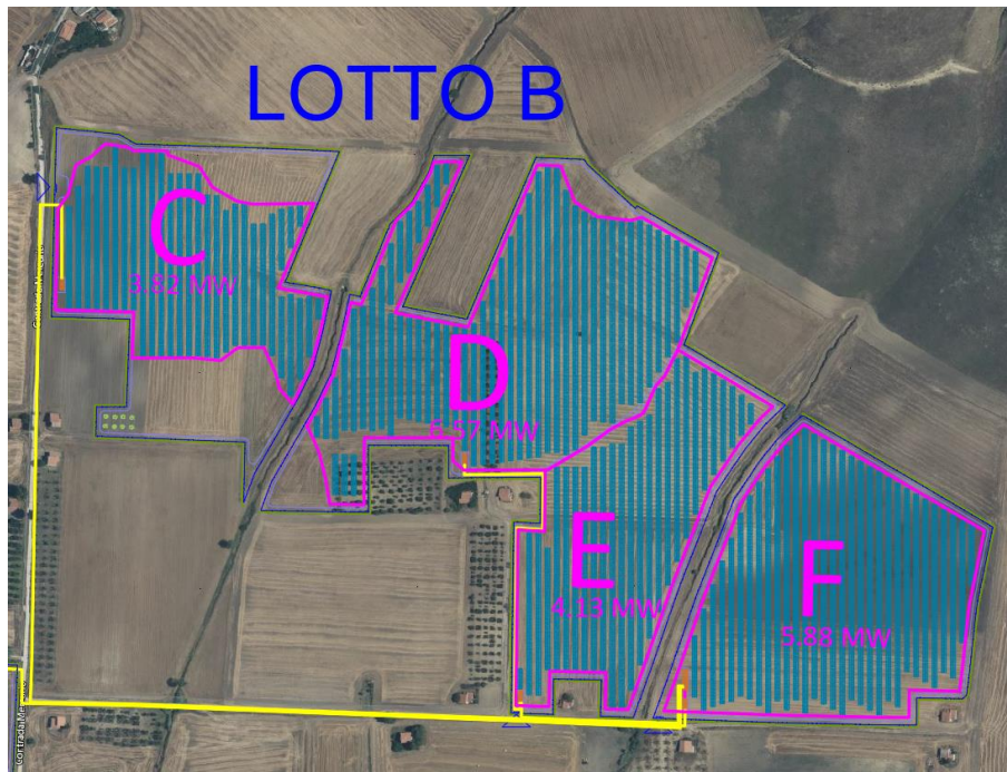
Figura 9 - Lotto B: collegamento entra-esce PS Sottocampo C e F, e Sottocampo D ed E
