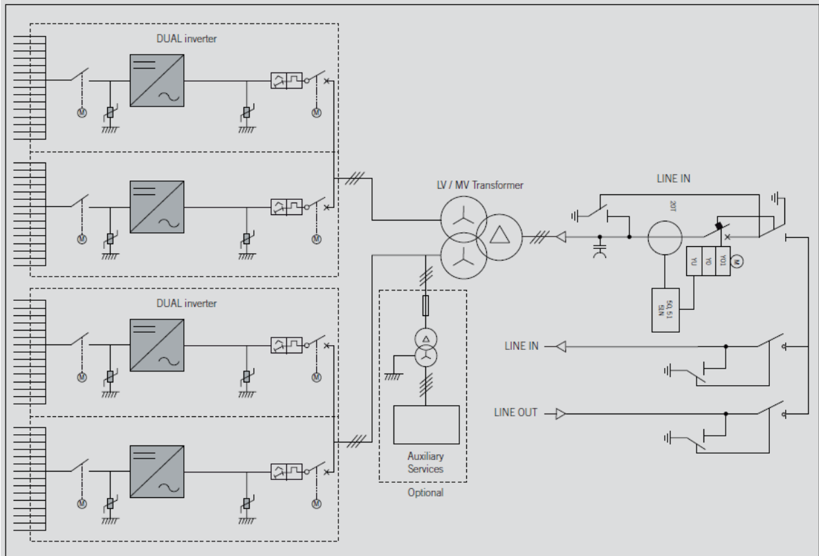
Figura 5 - Schema Elettrico Unifilare PS
