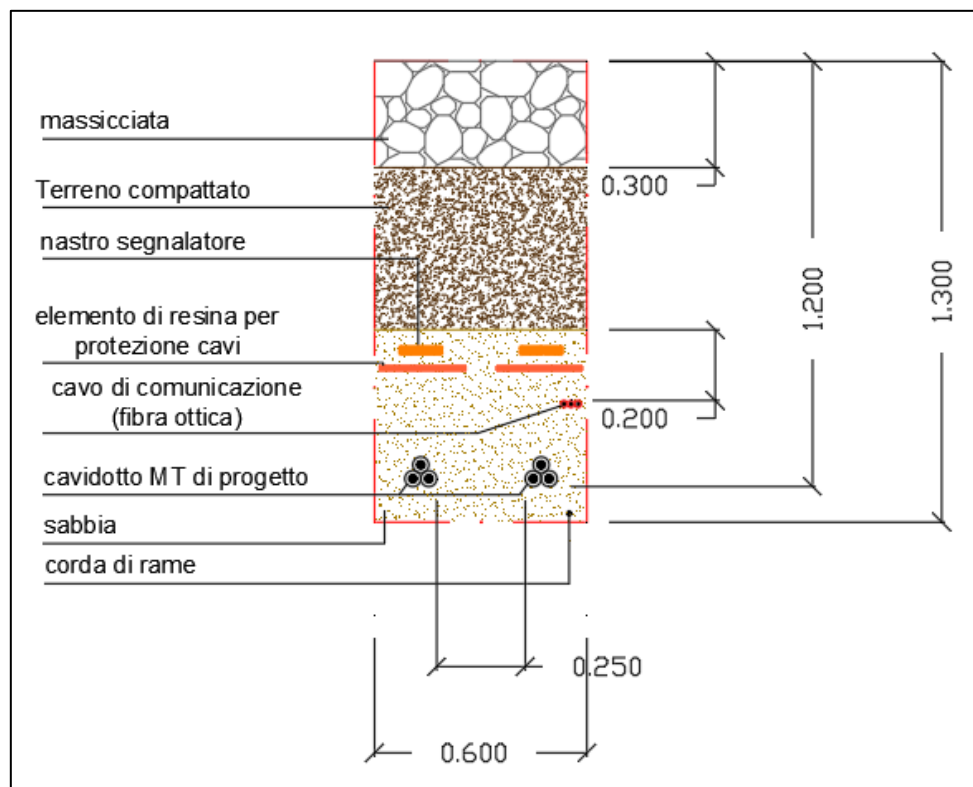
Figura 13 - Sezione Cavidotto doppia trina di cavi su Strada Bianca
