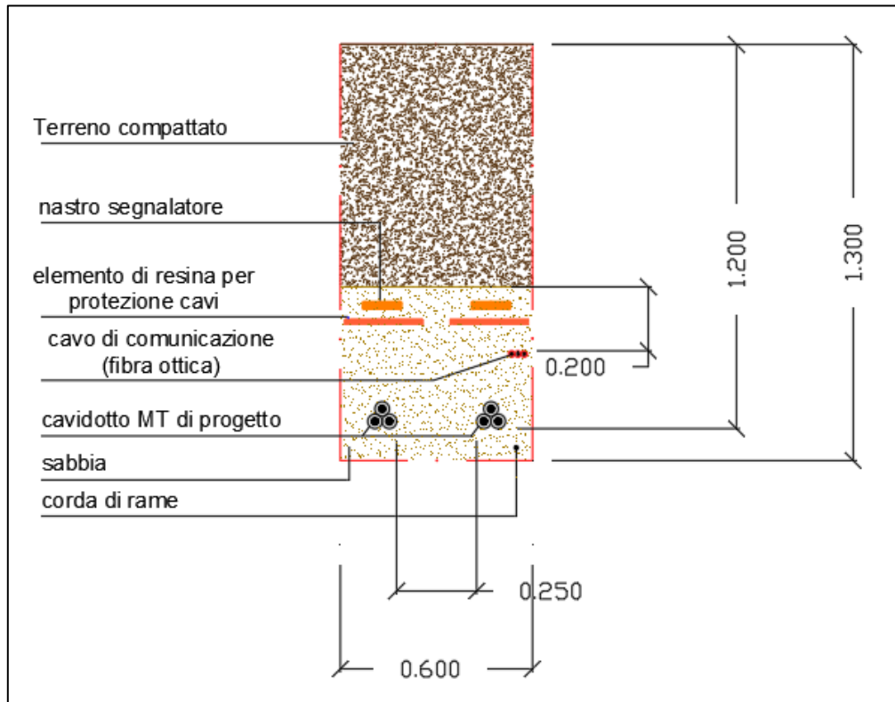
Figura 14 - Sezione Cavidotto doppia terna di cavi su Terreno
