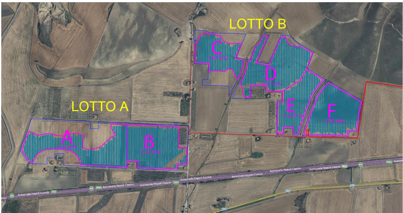
Figura 2 - Layout del campo Agro-fotovoltaico e suddivisione in sottocampi
