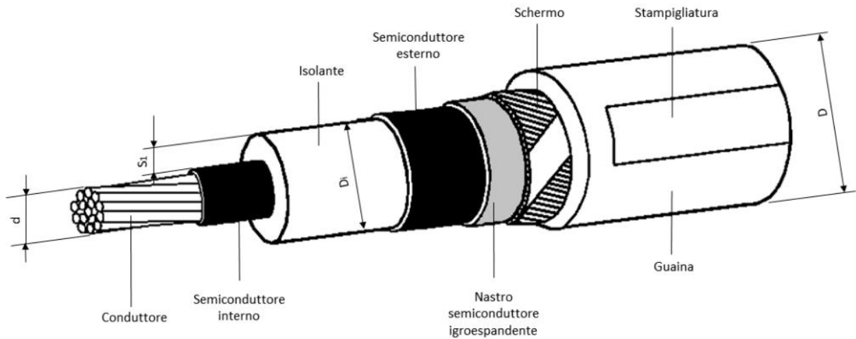
Figura 11 - Immagine indicativa del tipo di Cavo
