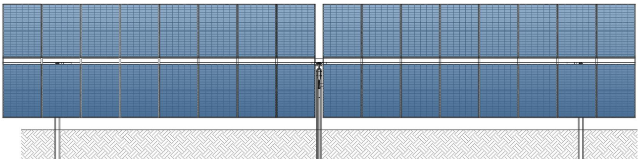
Figura 4 - Tracker 2P con Moduli FV: Vista Longitudinale
