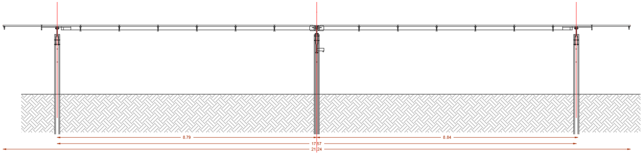
Figura 3 - Tracker 2P: Vista Longitudinale in condizione di riposo
