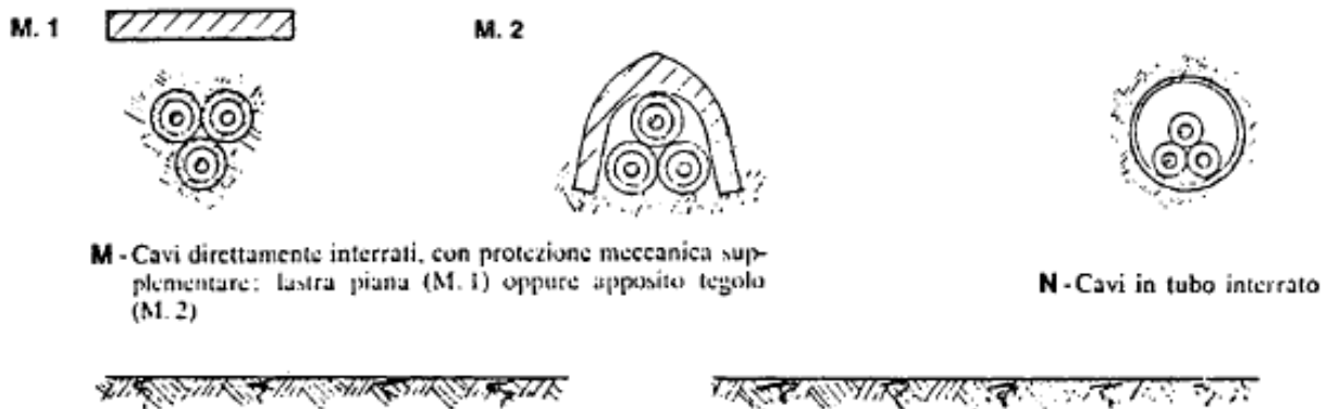
Figura 12 - Modalità di Posa (CEI 11-17)
