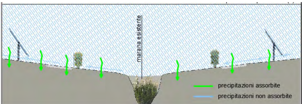
Figura 18 – Andamento qualitativo delle precipitazioni (assorbimento e dilavamento)
