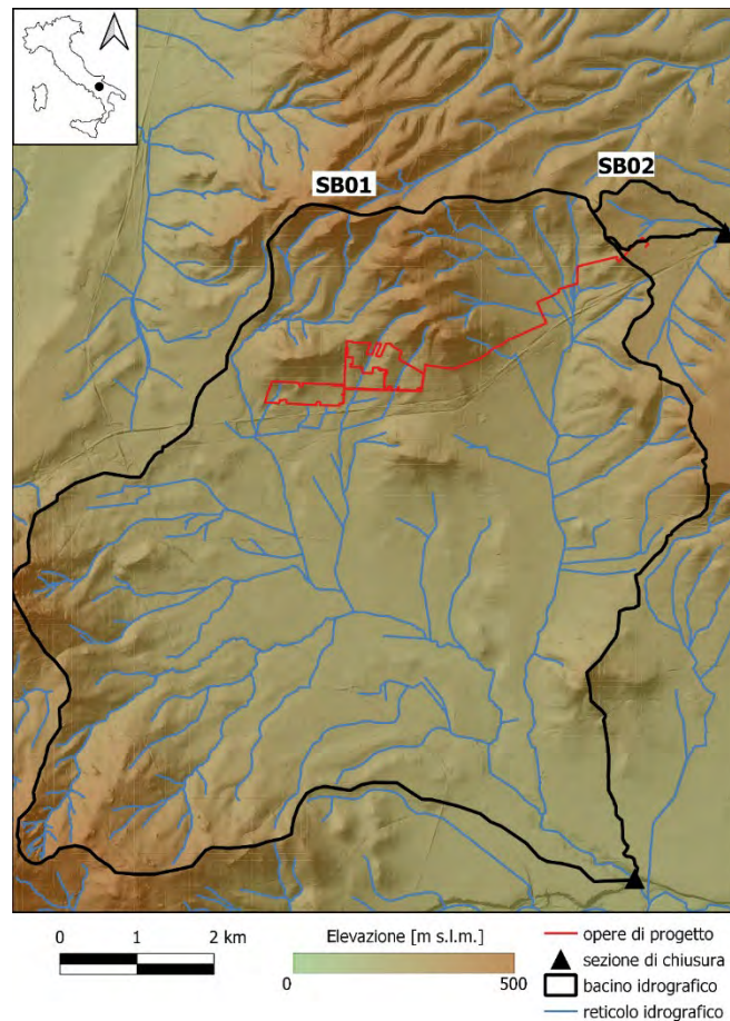
Figura 15 - Inquadramento dei sotto-bacini idrografici riguardanti le opere di progetto su modello digitale del terreno
