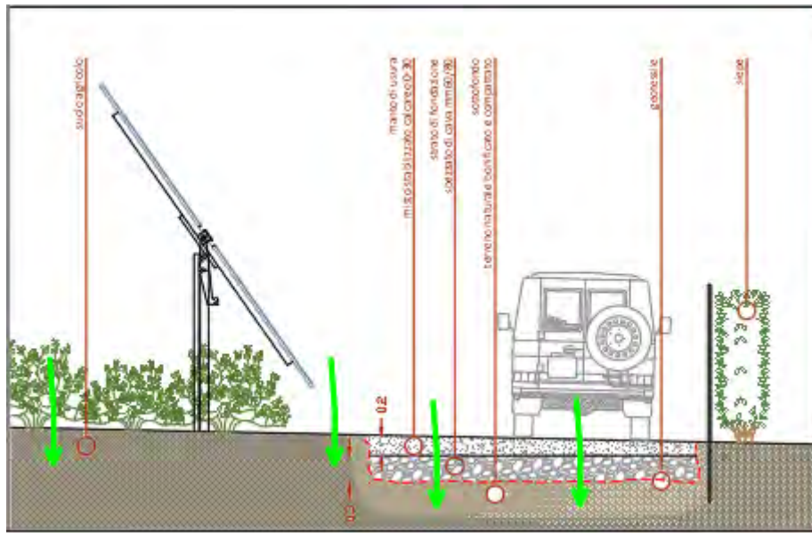
Figura 19 – Viabilità interna al parco: assorbimento delle precipitazioni
