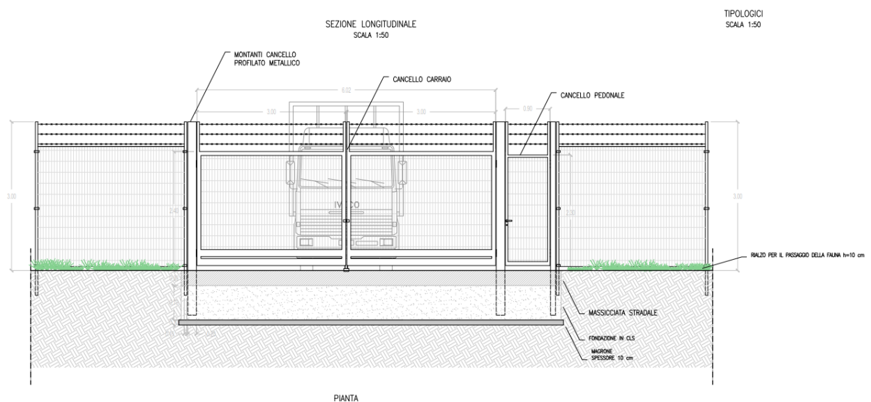
Figura 5.1: Tipico recinzione
