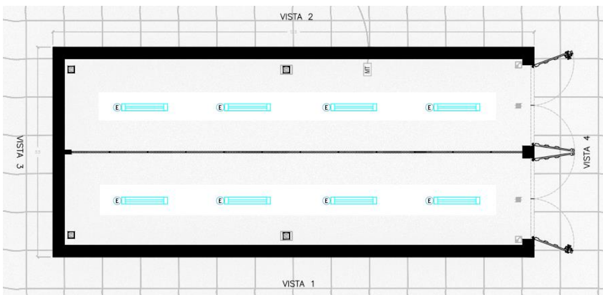
Figura 4.3 – Posizionamento plafoniere magazzino.
