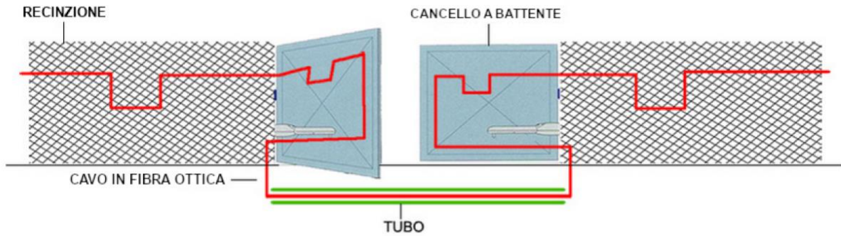
Figura 4.9 – Schema di installazione cavo in fibra ottica su recinzione.
