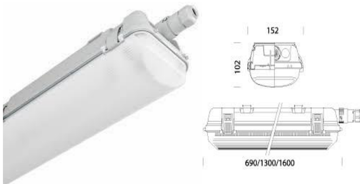
Figura 4.6 – Plafoniera LED tipo ECHO
