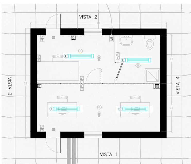
Figura 4.4 – Posizionamento plafoniere Cabina Uffici.
