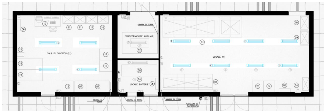
Figura 4.5 – Posizionamento plafoniere Cabina BT/MT.
