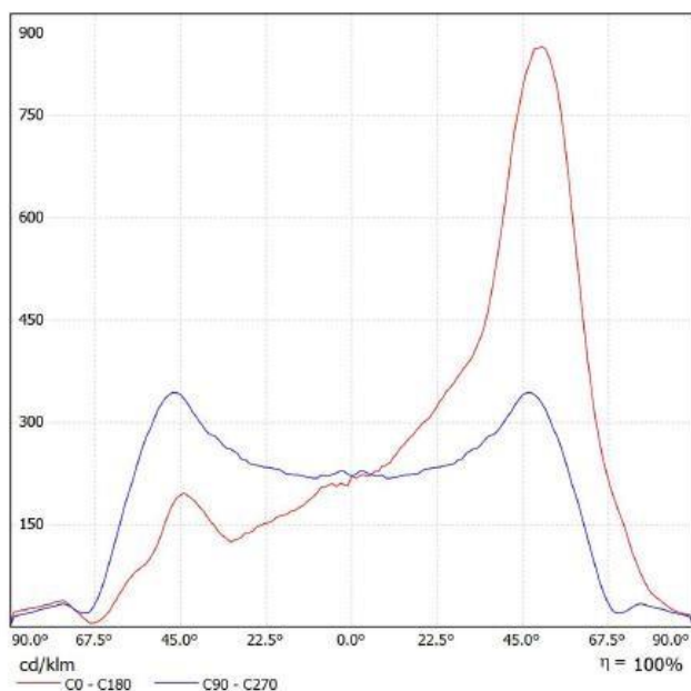
Figura 4.2 – Fotometria Lampada: Disano 1151 Indio – LED asimmetrico Disano 1151 48 led CLD CELL grafite
