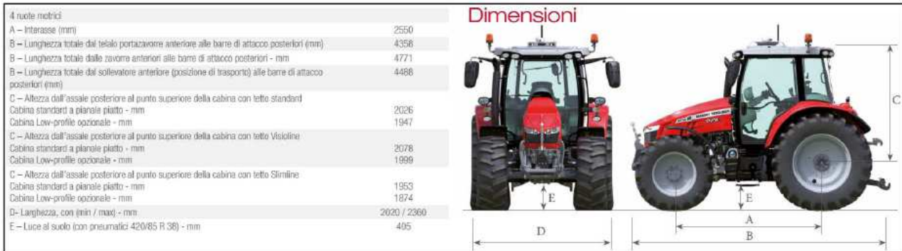
Figura 6.6: Dimensioni di una trattrice gommata ideale per la gestione dell'azienda (Fonte: Massey-Ferguson)
