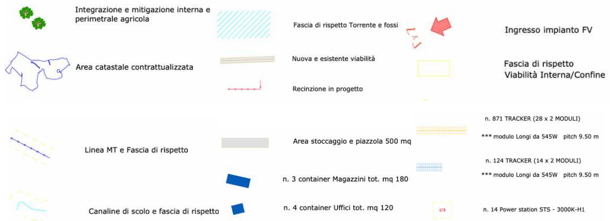
Figura 3.1: Layout di progetto
