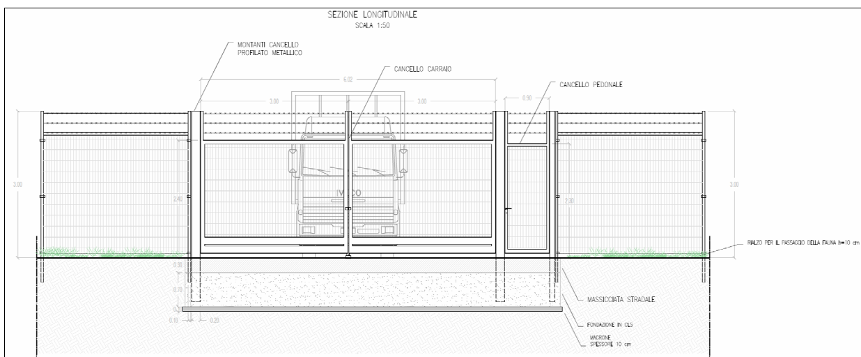
Figura 3.4: Particolare accesso
