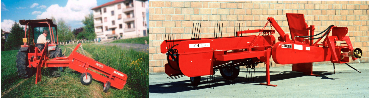
Figura 6.10: ranghinatore per argini e fossati risolve l’annosa e faticosa rastrellatura manuale dell’erba nei fossi, nei canali e sugli argini, ma è adatto anche alle normali operazioni in piano (Foto: Cucchi)
