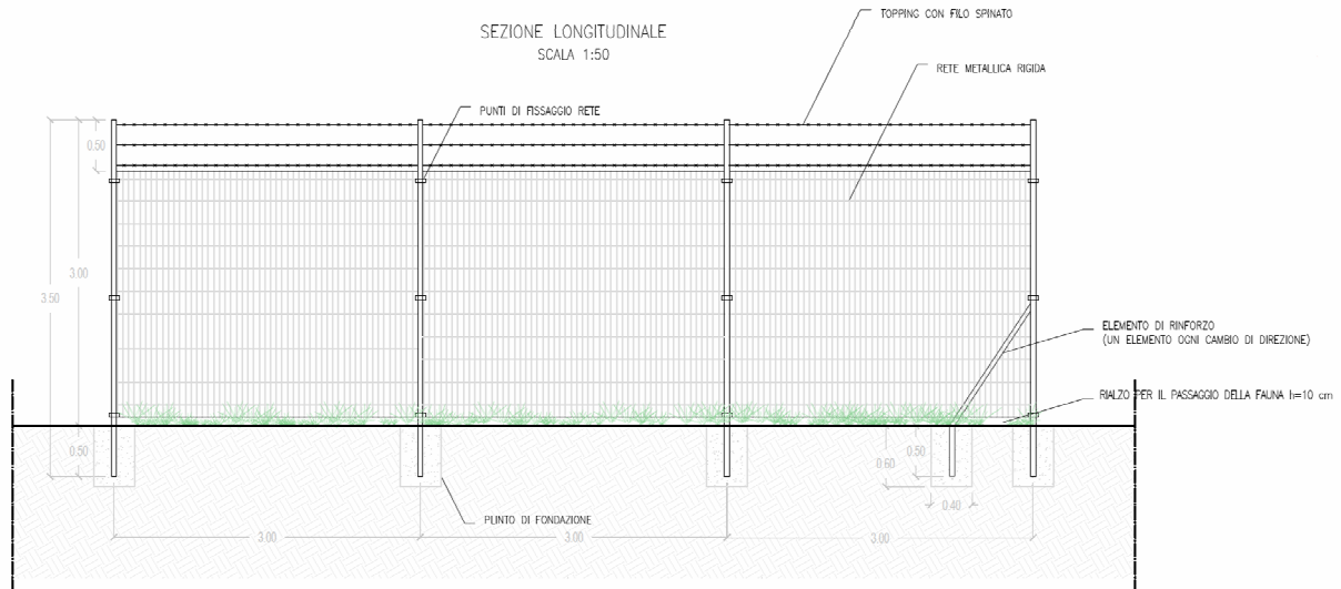
Figura 3.3: Particolare recinzione
