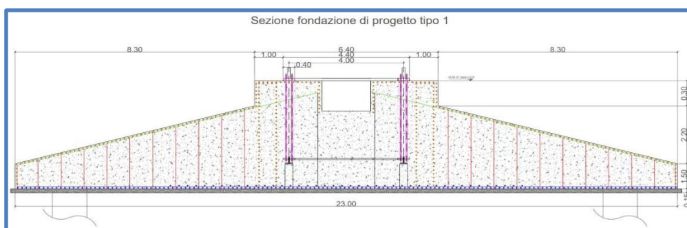
Figura 6 - Tipologia fondazione
