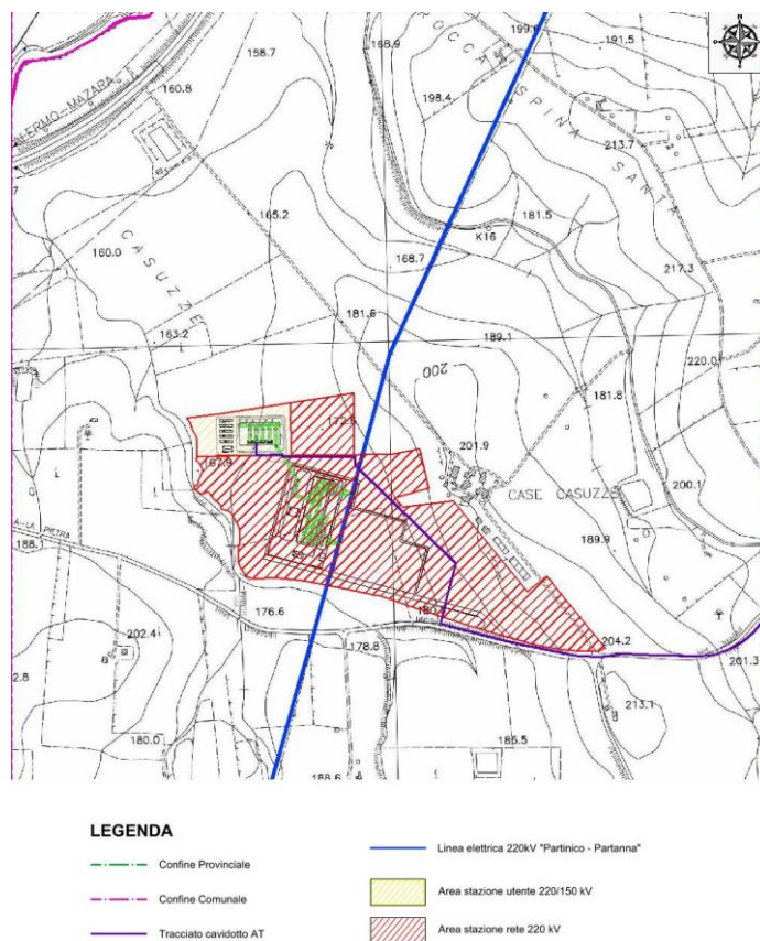
Fig. 8 – Layout stazione di connessione su CTR
