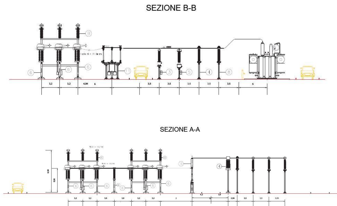
Fig. 11 - Profili stazione rete – Utente
