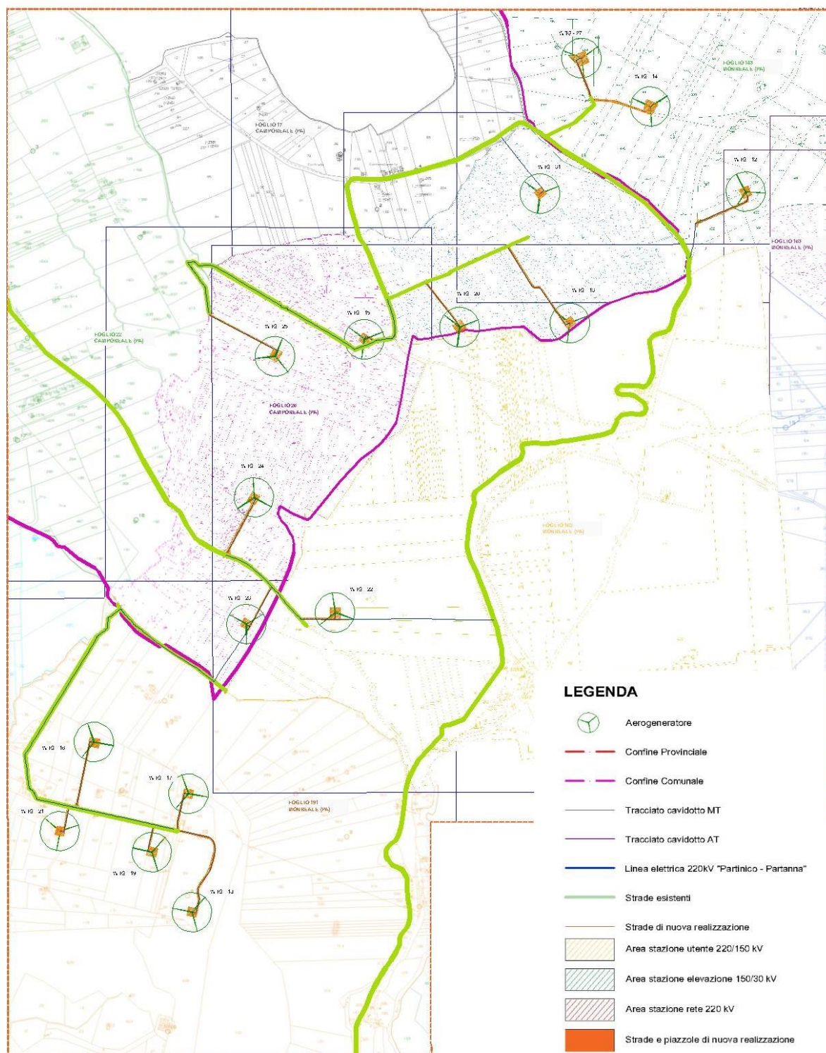
Figura 4 B – Layout su Catastale dell’area d’impianto ricadente nelle Contrade Montagnola, Macellarotto, Borrachine
