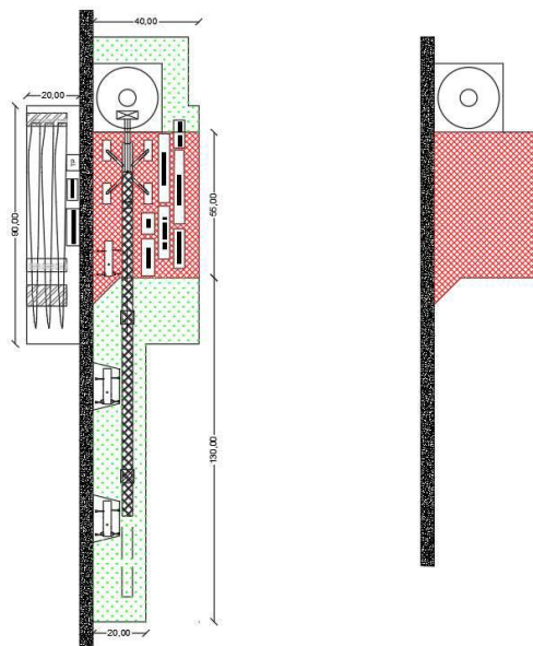
Figura 7 - Piazzola aerogeneratore durante la fase di montaggio (a sinistra) e a conclusione delle lavorazioni (destra)
