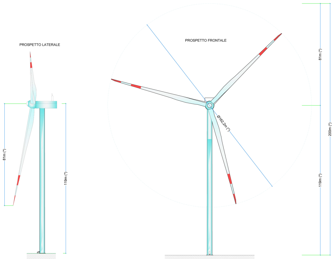
Fig. 18 - Rappresentazione grafica dell'aerogeneratore
