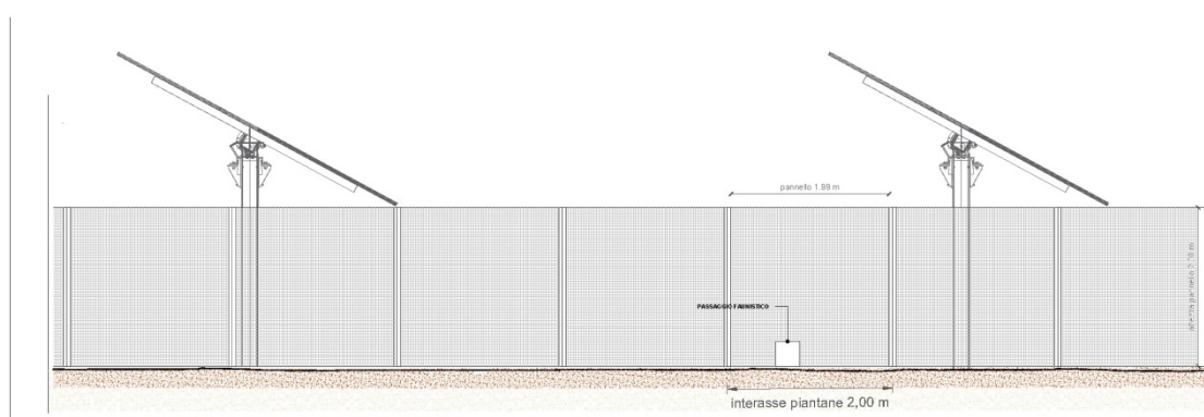
Figura 24 – Prospetto recinzione perimetrale senza mitigazione
