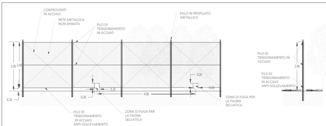
Tipologico recinzione
