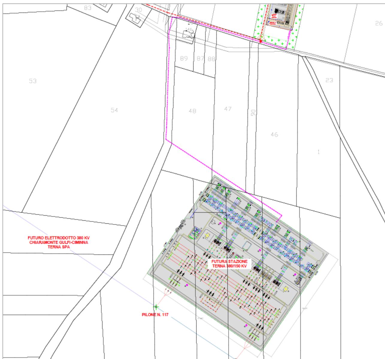
Tracciato elettrodotto AT interrato su planimetria catastale (Tavola FR-RADDUSA-AFV-PD-D-5.1.4.0)
