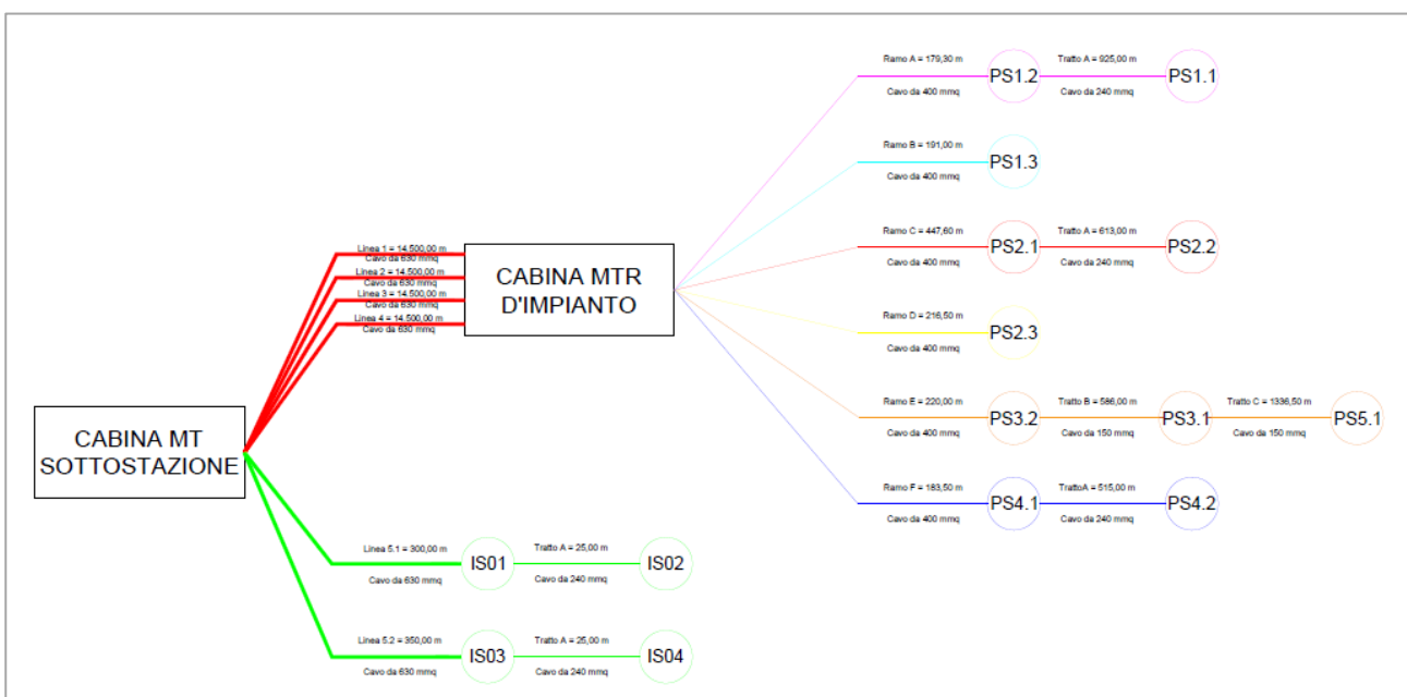
Configurazione linee e rami (tratto da Tavola R-RADDUSA-AFV-PD-D-3.2.7.0 - SCHEMA ELETTRICO UNIFILARE MT)
