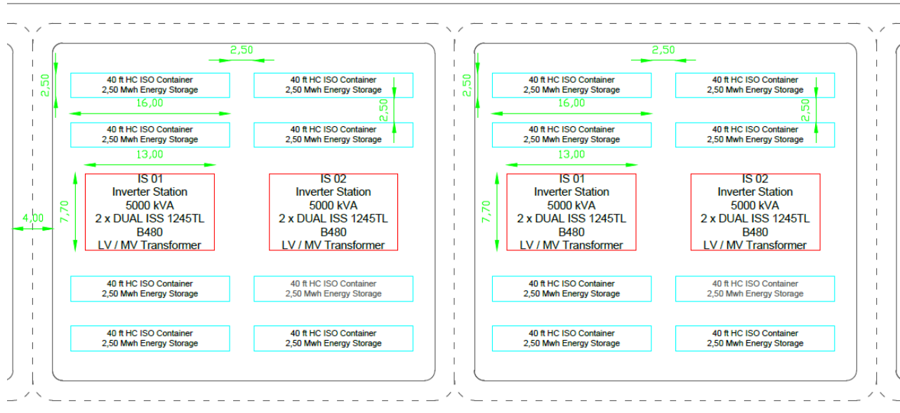
Configurazione ESS – Sezioni 2 e 3 “Raddusa”
