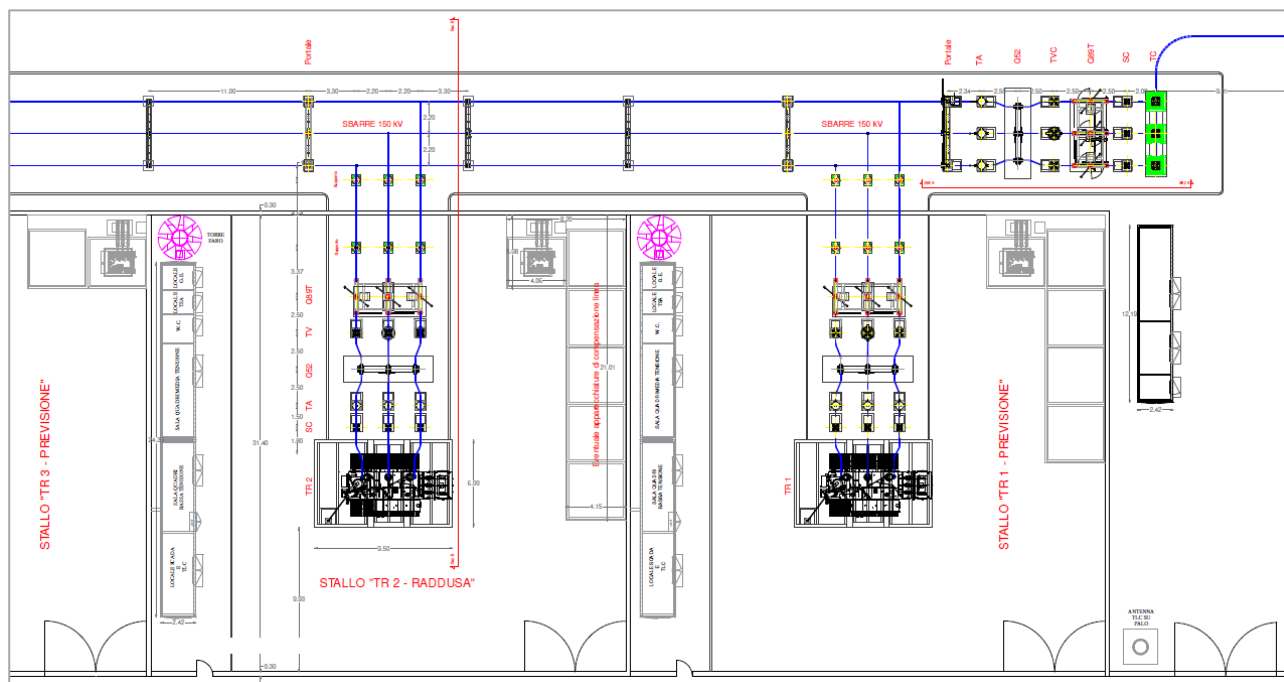
Pianta elettromeccanica della SSE - Stallo MT/AT "TR2 – Raddusa" (Tavola FR-RADDUSA-AFV-PD-D-5.2.2.0)
