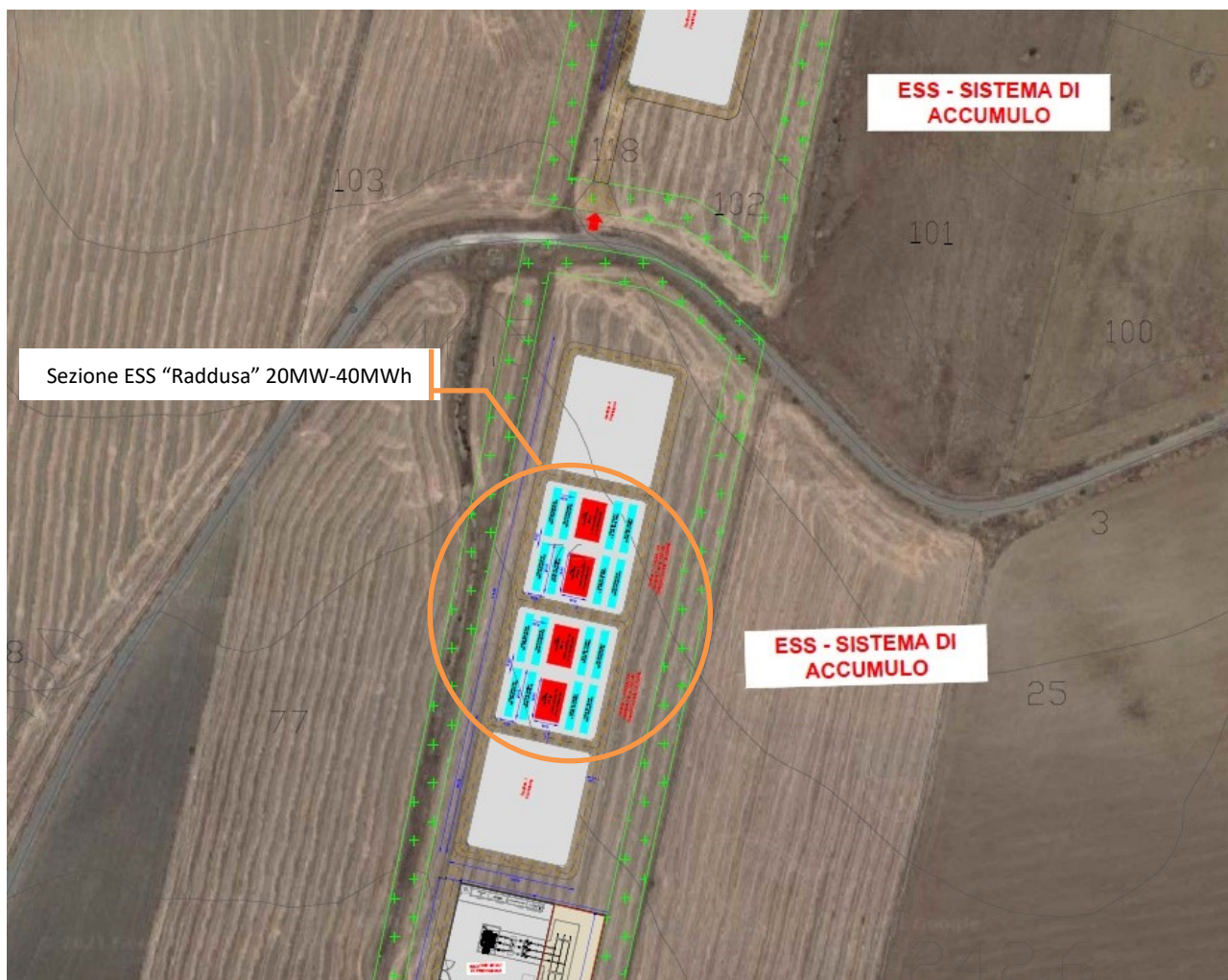
Lay-out Sistema di Accumulo (ESS) – Sezione 2 “Raddusa”
