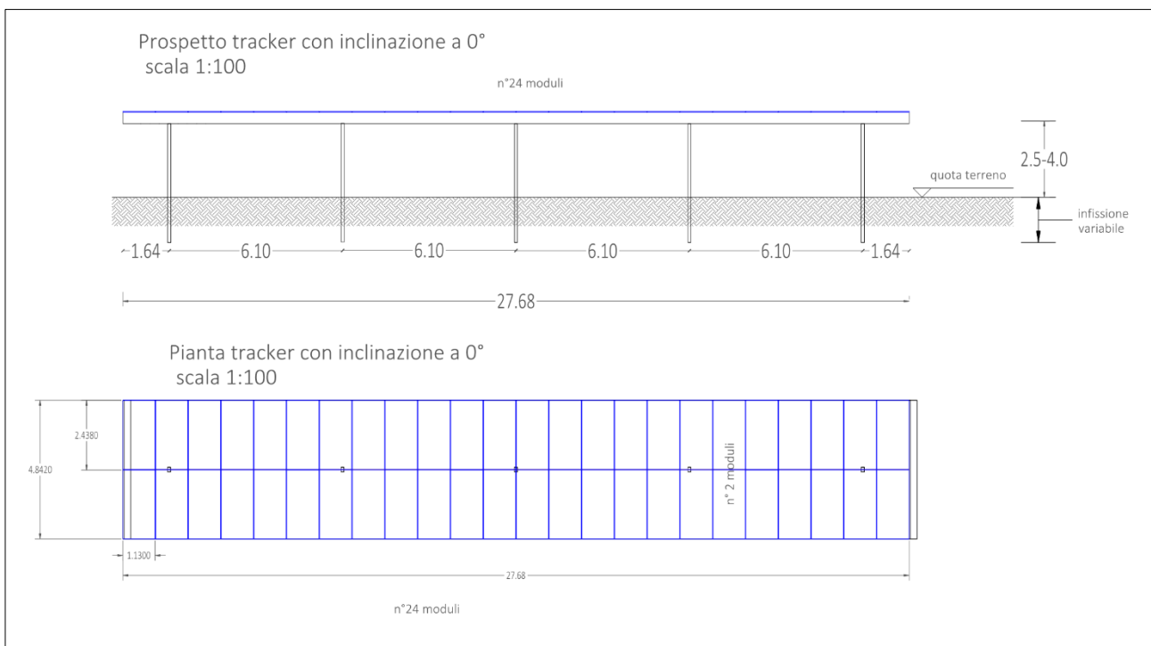
Tipologico struttura sostegno moduli – piante e prospetti della configurazione 2P24 da 48 moduli (Tavola FR-RADDUSA-AFV-PD-D-3.3.1.0-r0A-R00)
