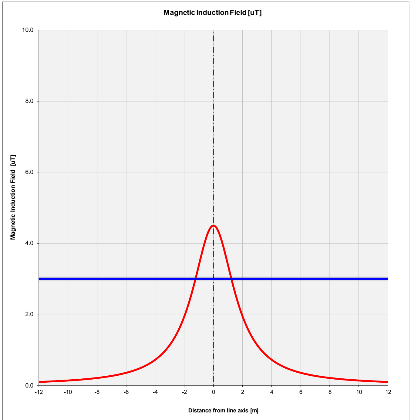
Figura 6: Andamento dell'induzione magnetica prodotta dalla linea in cavo AT
