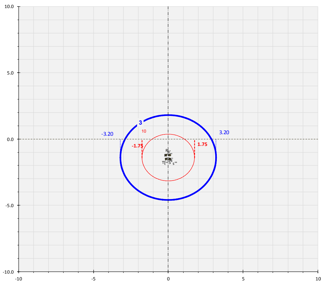
Figura 5: Curve di equilivello per il campo di induzione magnetica generato dalla linea MT (Sezione a quattro terne MT)
