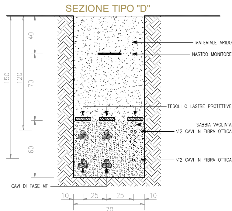
Figura 2: Sezioni tipiche di posa della linea in cavo su strade sterrate
