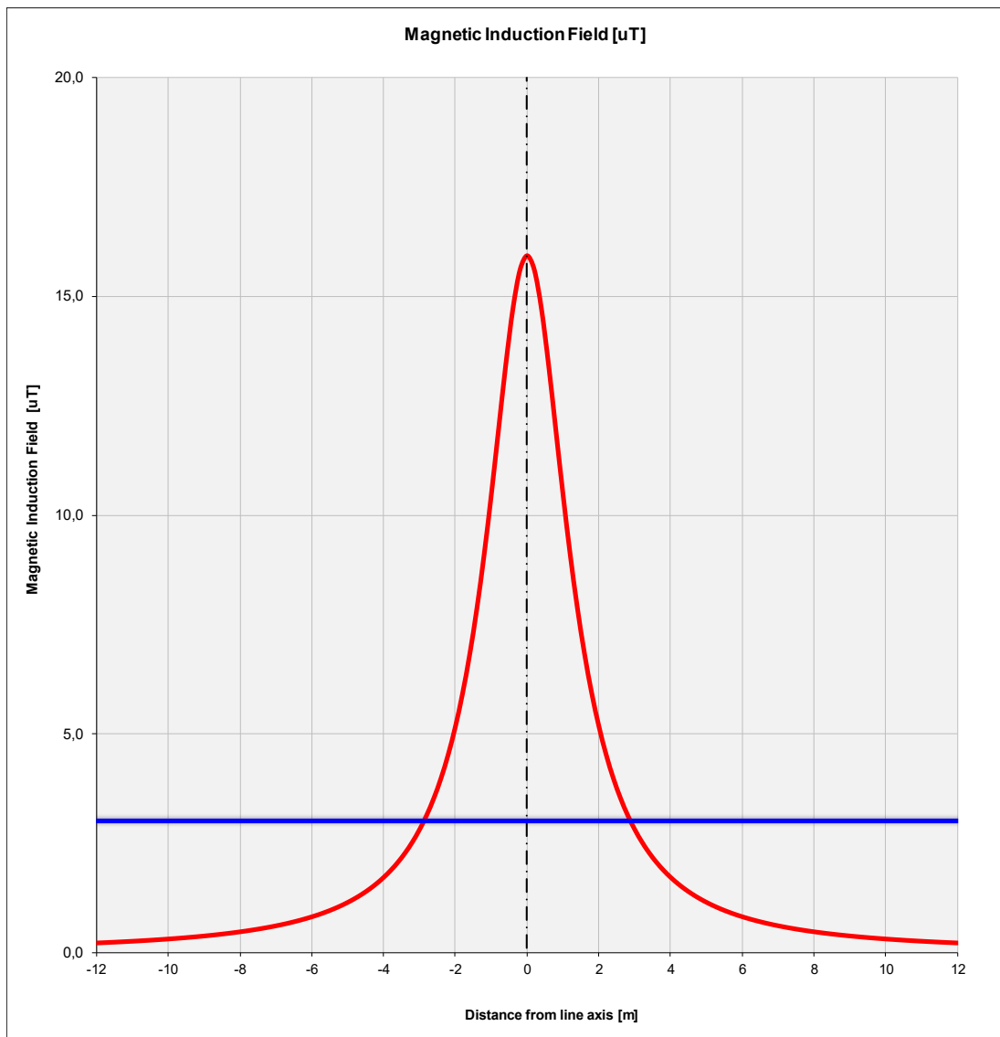
Figura 4: Andamento dell'induzione magnetica prodotta dalla linea in cavo per la sezione (quattro terne MT)
