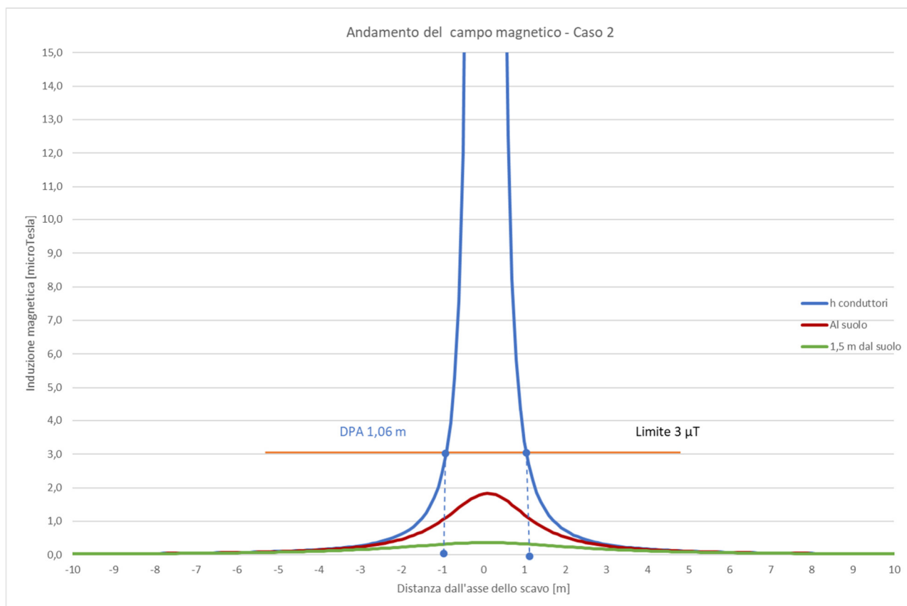
Figura 2: Andamento del campo magnetico in funzione della distanza dall'asse dei conduttori in forma grafica relativa CASO 2.
