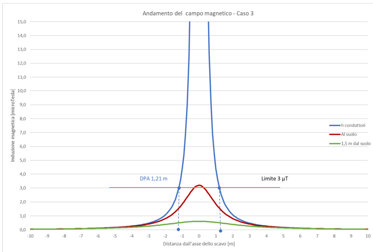
Figura 3: Andamento del campo magnetico in funzione della distanza dall'asse dei conduttori in forma grafica relativa CASO 3.
