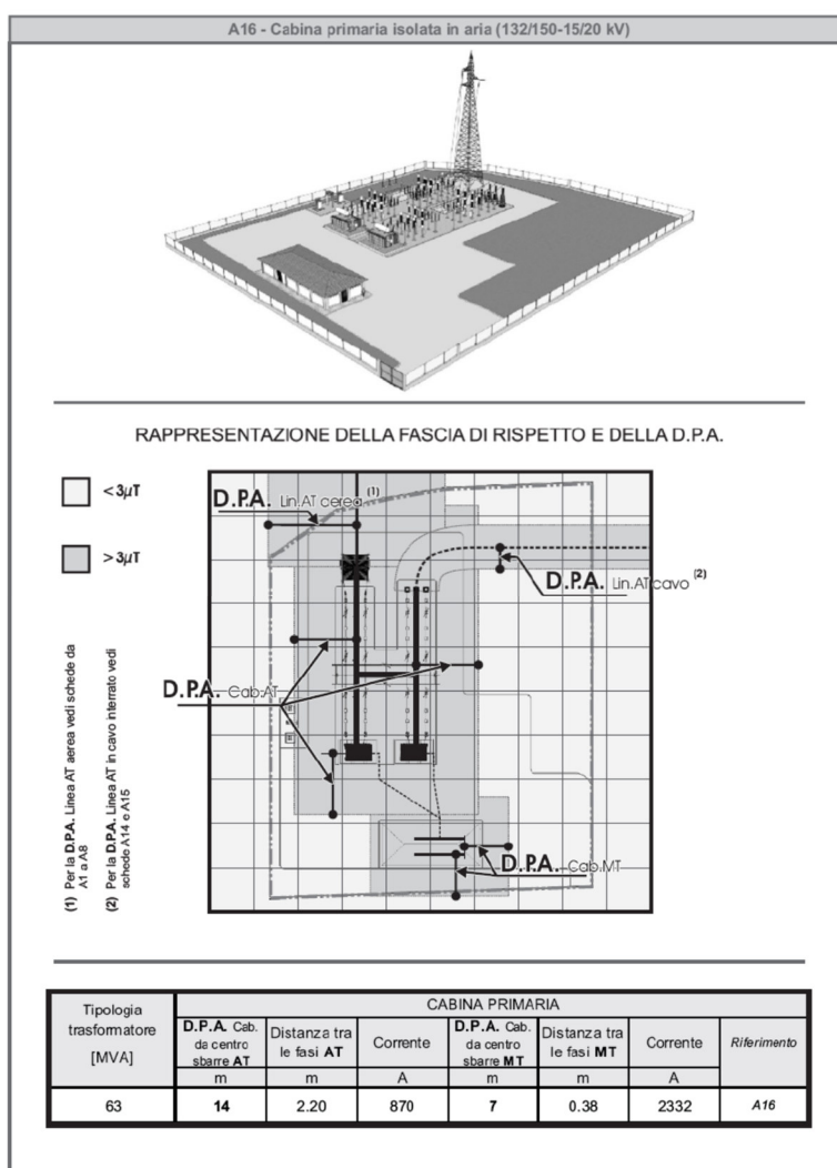
Figura 8: Esempio di fasce di rispetto relative ad una cabina primaria
