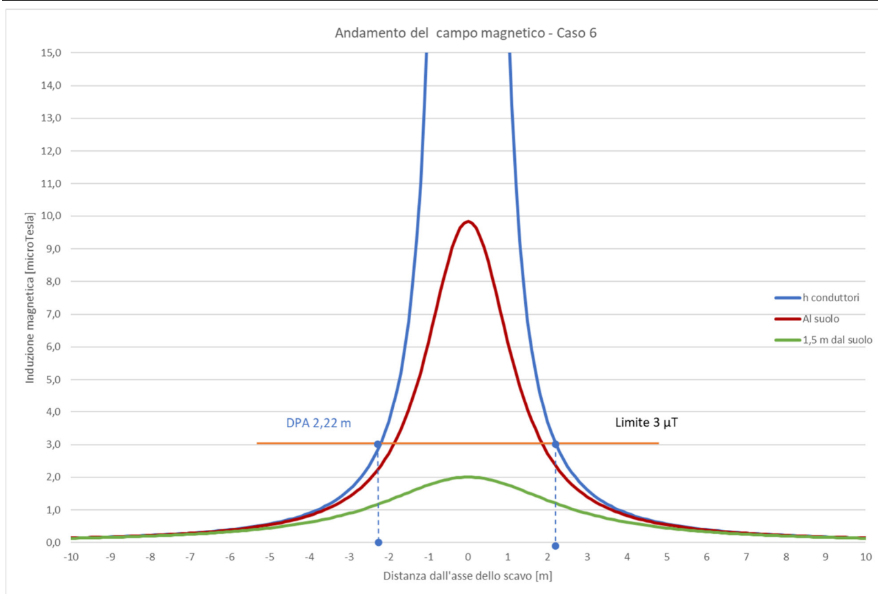
Figura 6: Andamento del campo magnetico in funzione della distanza dall'asse dei conduttori in forma grafica relativa CASO 6.
