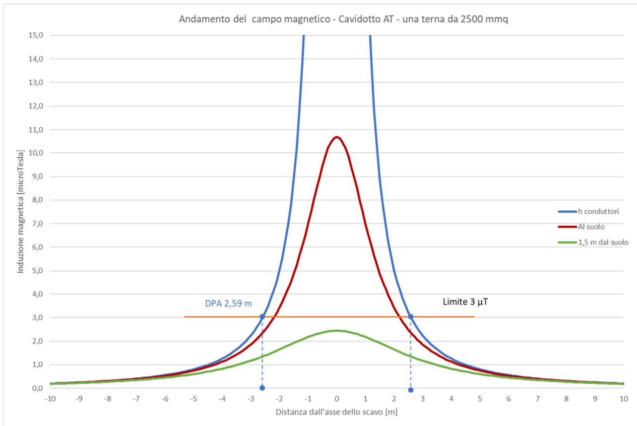
Figura 9: Andamento del campo magnetico in funzione della distanza dall'asse dei conduttori in forma grafica relativa al cavidotto AT
