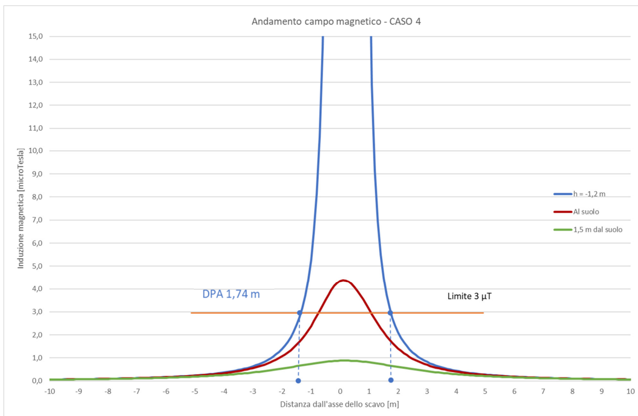
Figura 4: Andamento del campo magnetico in funzione della distanza dall'asse dei conduttori in forma grafica relativa CASO 4.
