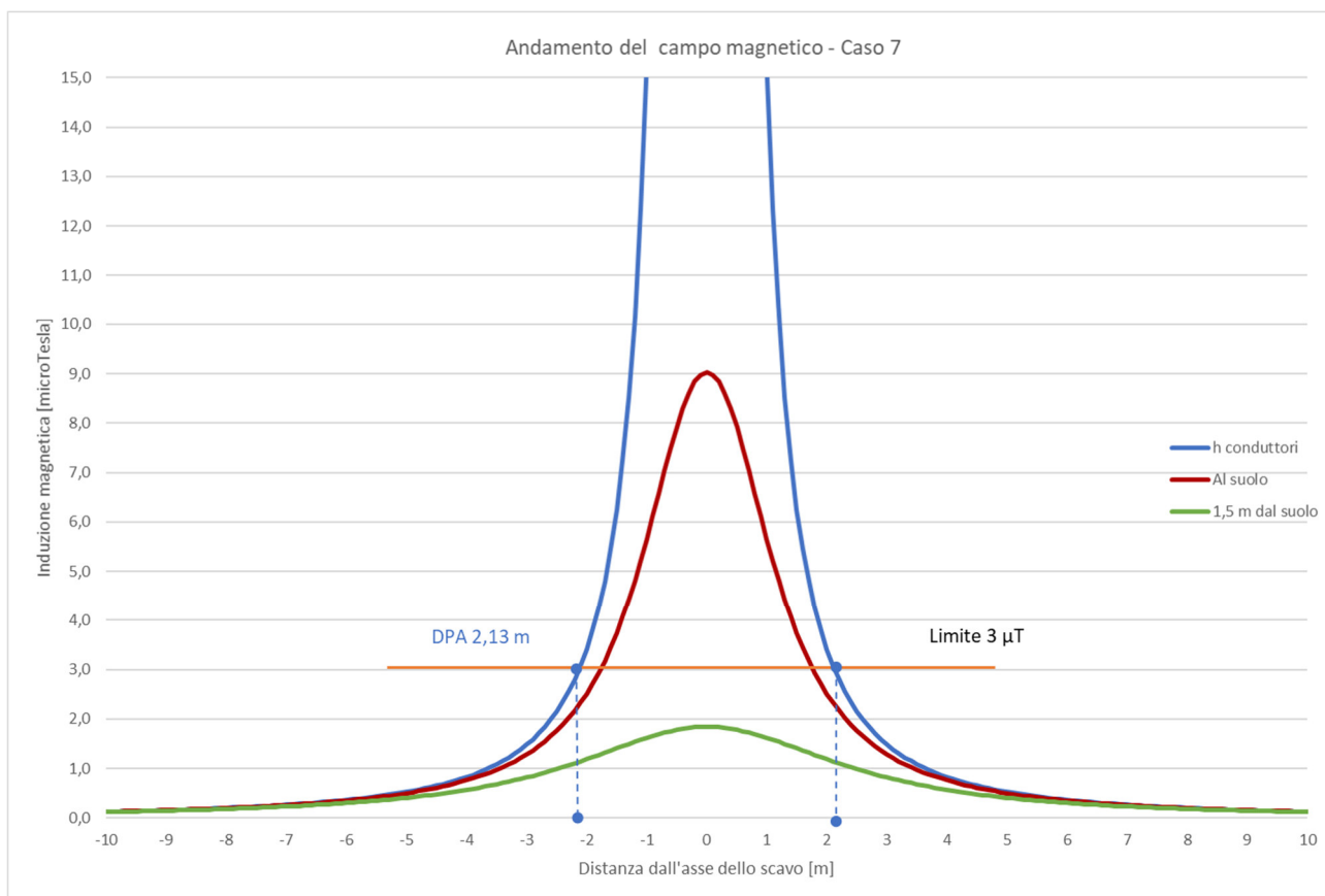
Figura 7: Andamento del campo magnetico in funzione della distanza dall'asse dei conduttori in forma grafica relativa CASO 7.
