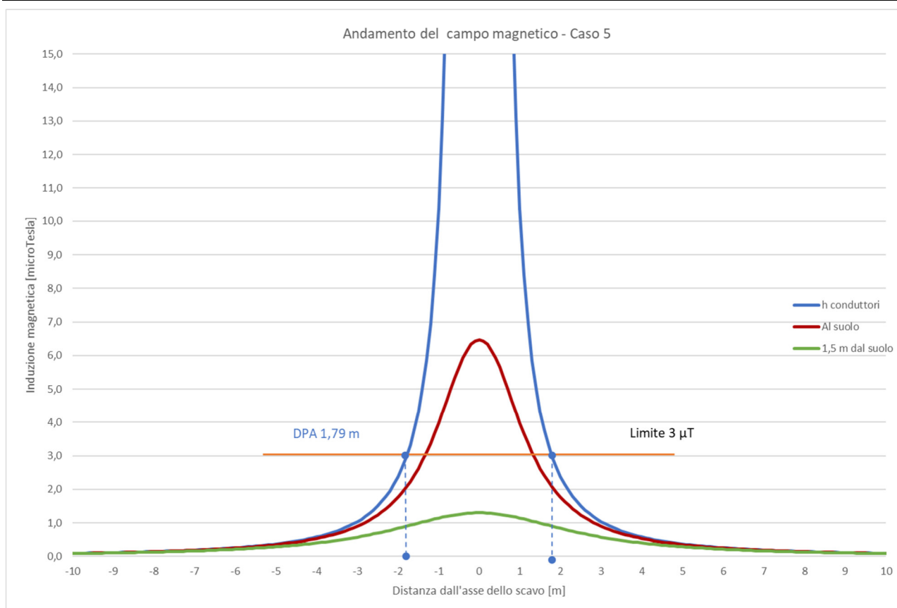
Figura 5: Andamento del campo magnetico in funzione della distanza dall'asse dei conduttori in forma grafica relativa CASO 5.
