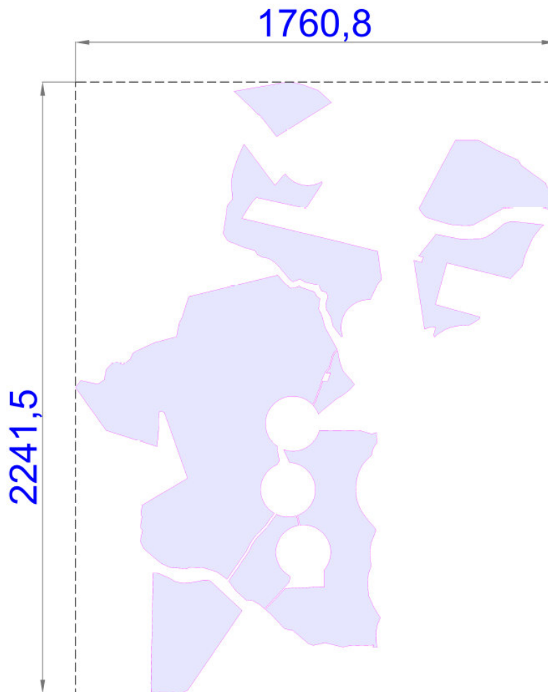
Fig. 3 – Modello geometrico del Generatore fotovoltaico
