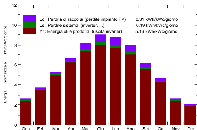
Produzione normalizzata (per kWp installato): Potenza nominale 37613 kWc
