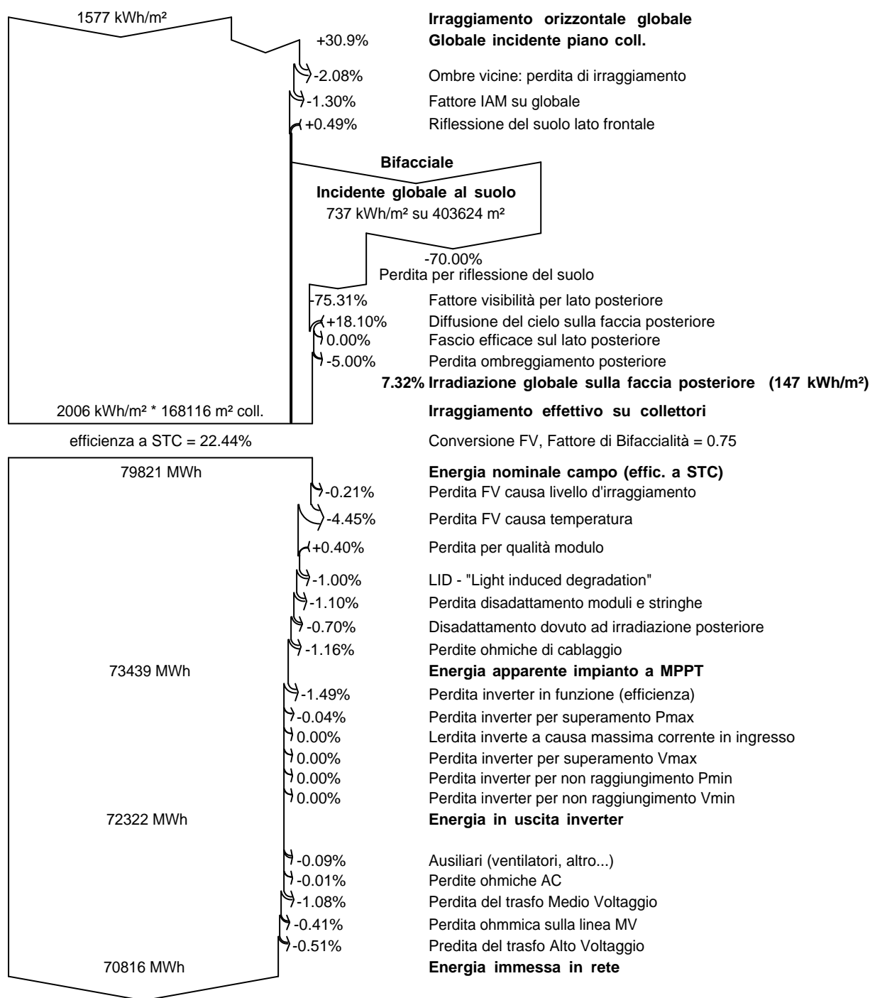
Diagramma perdite sull'anno intero
