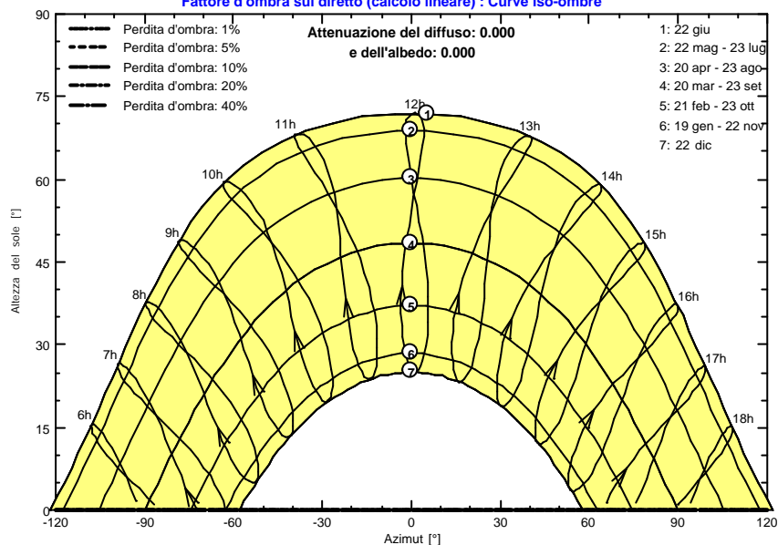
Diagramma iso-ombre
