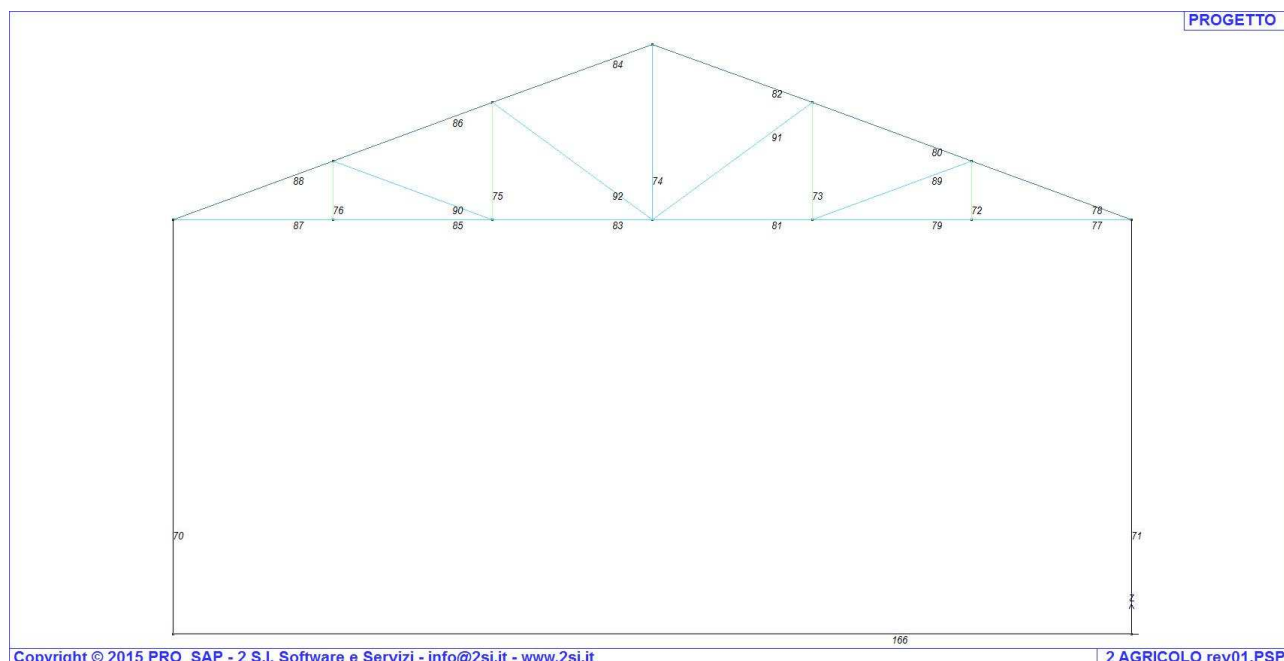
Figura 36: Modello 2D dell'edificio agricolo
