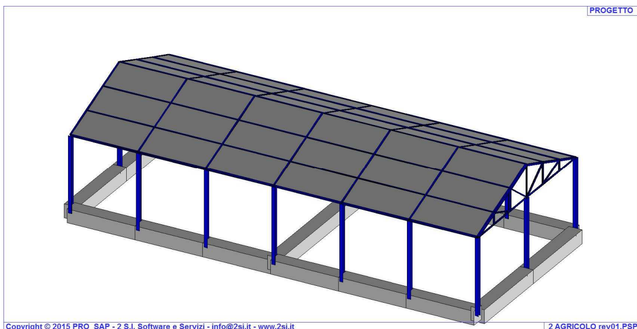
Figura 33: Schema tipo struttura
