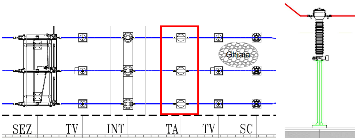
Figura 21: Tipico trasformatore di corrente – vista prospettica e planimetrica
