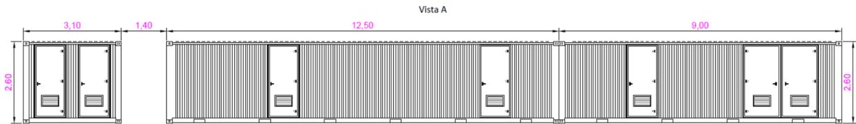
Figura 25: Vista frontale Container
