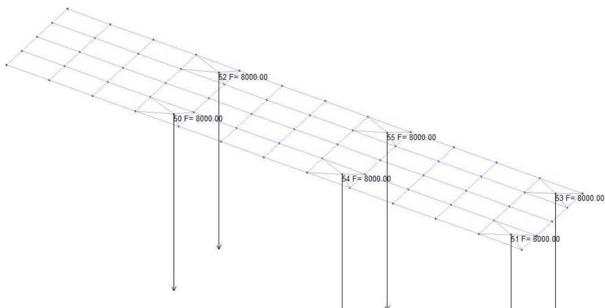
Figura 31: carichi concentrati nodali - scarichi al piede
