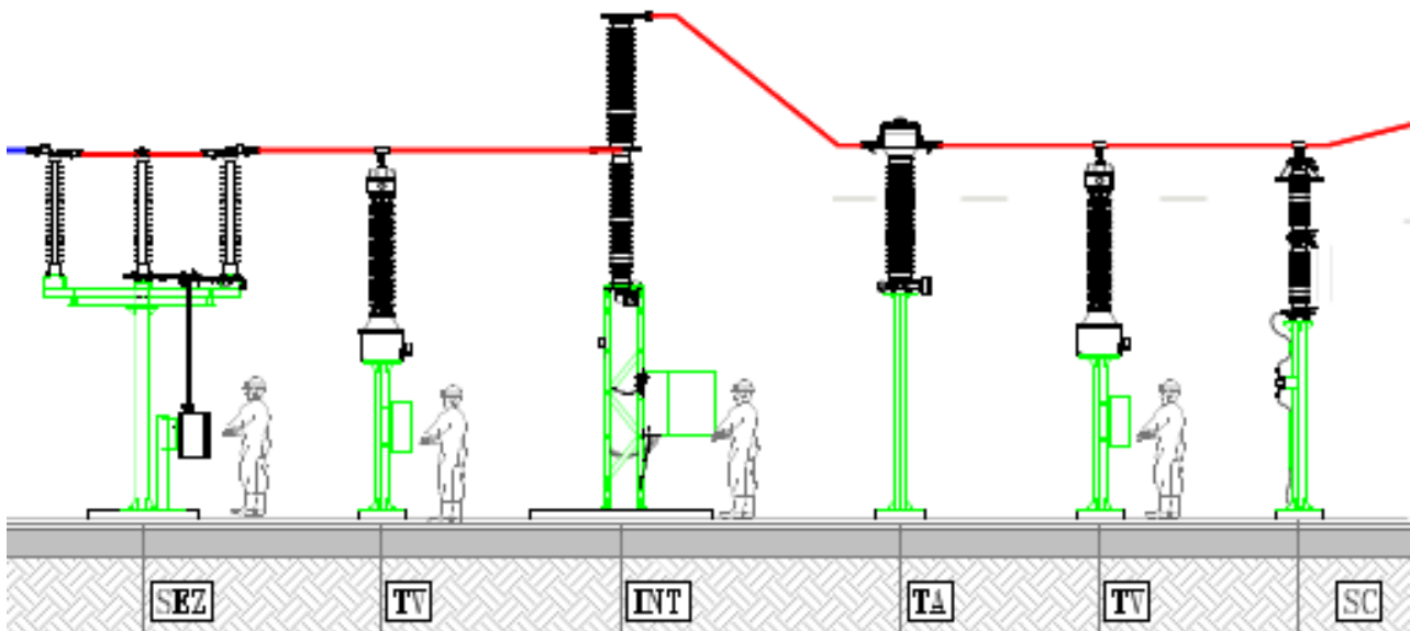
Figura 16: vista sezione elettromeccanica Apparecchiature AT
