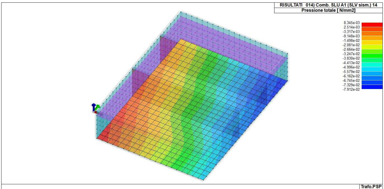
Figura 9: RIS_PRESSIONI_014_Comb. SLU A1 (SLV sism.) 14
