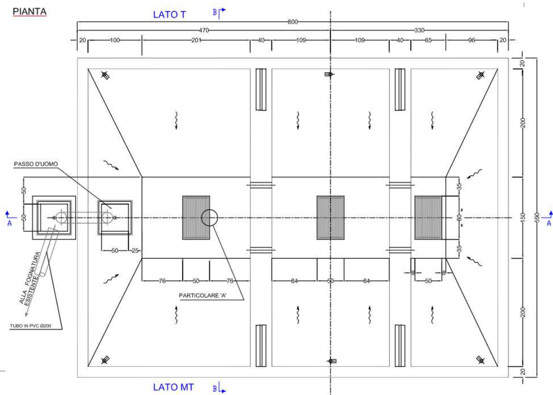
Figura 1: Pianta fondazione trasformatore
