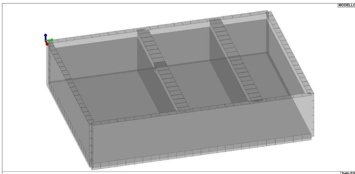
Figura 3: Modello FEM (senza soletta di copertura) – Vista 3D
