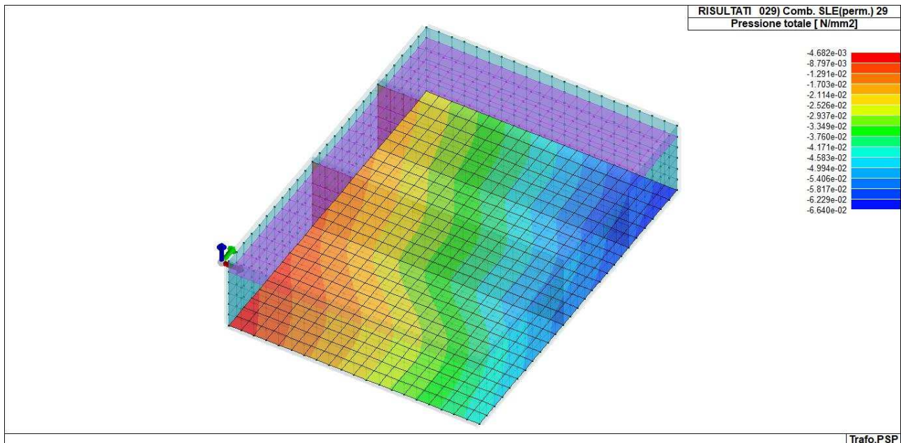
Figura 15: ANDAMENTO DEI CARICHI AL SUOLO
