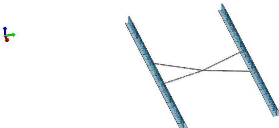
Figura 4: Modello FEM – Vista dei soli elementi trave
