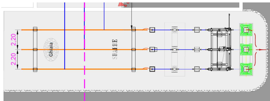
Figura 23: vista planimetrica sistema Sbarre Condivise
