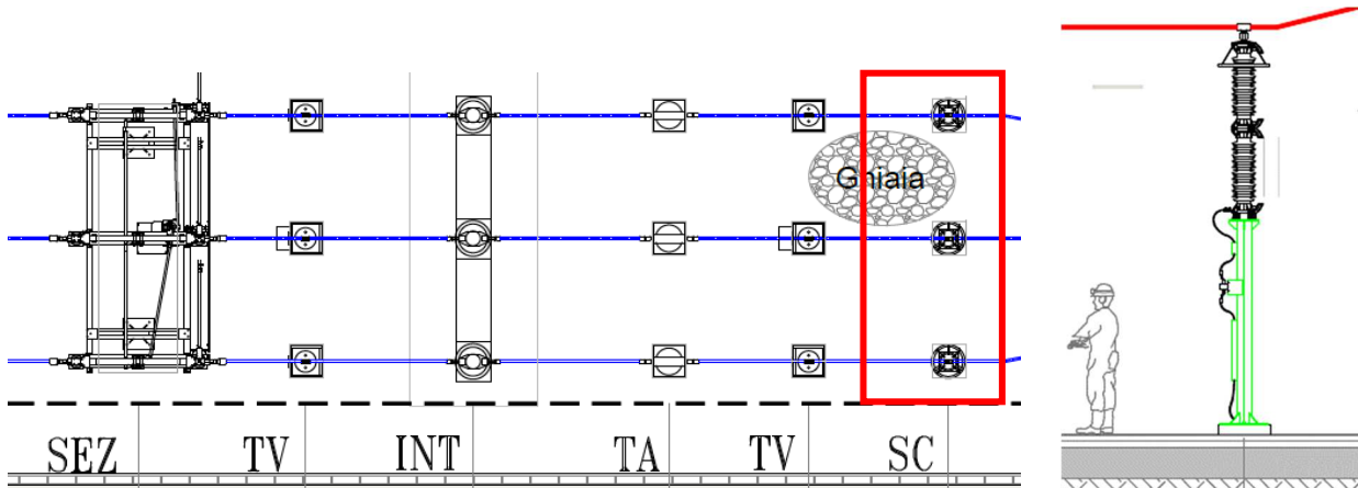
Figura 22: Tipico scaricatore di sovratensione – vista prospettica e planimetrica
