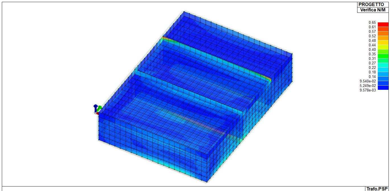
Figura 13: Verifiche elementi shell N/M
