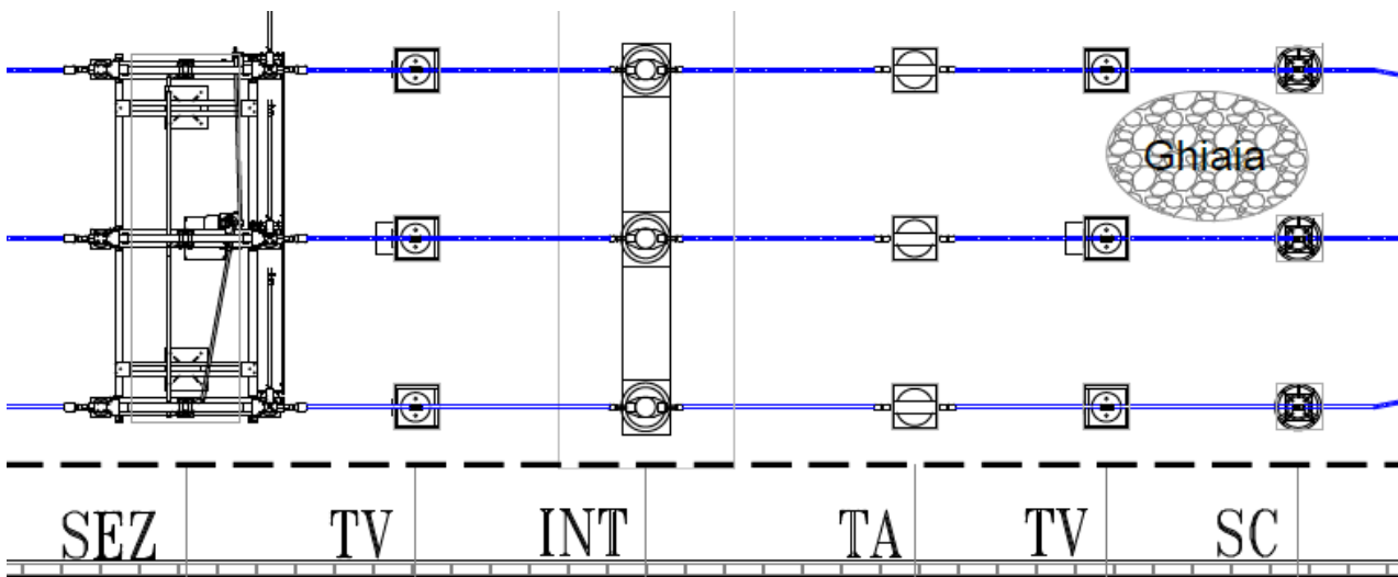
Figura 17: planimetria elettromeccanica apparecchiature AT
