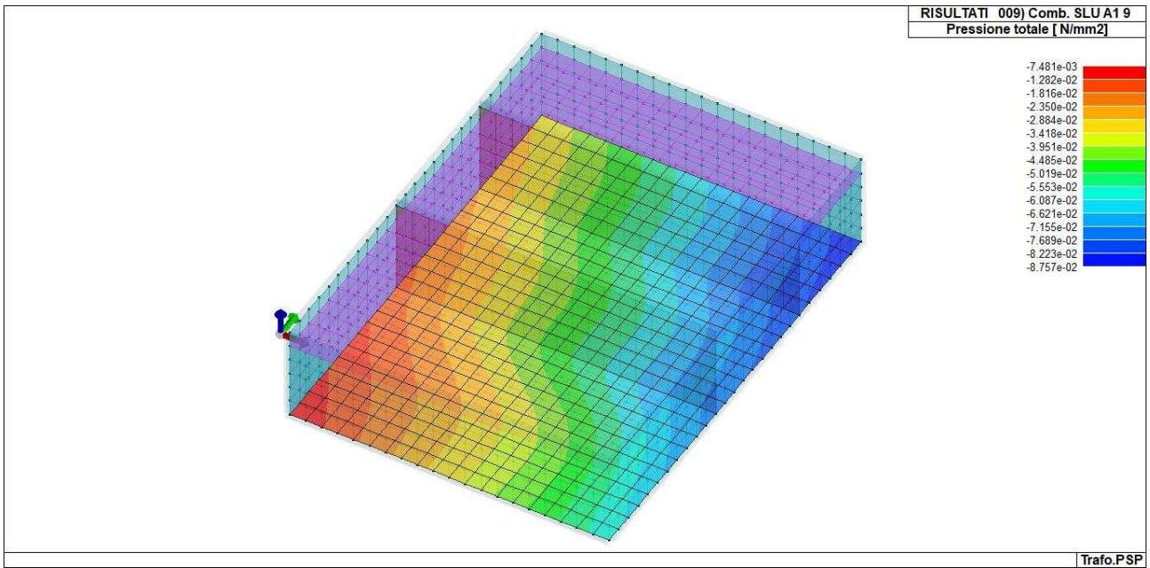
Figura 8: RIS_PRESSIONI_009_Comb. SLU A1 9
