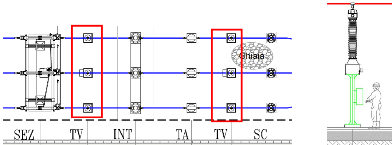
Figura 20: Tipico Trasformatore di tensione – vista prospettica e planimetrica
