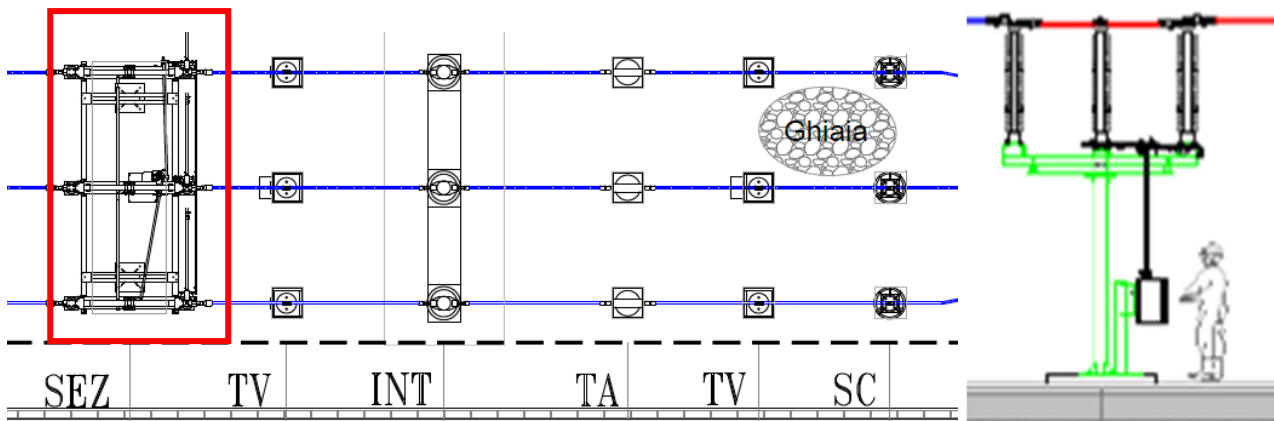
Figura 18: Tipico sezionatore tripolare – vista prospettica e planimetrica
