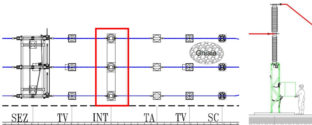
Figura 19: Tipico interruttore tripolare – vista prospettica e planimetrica
