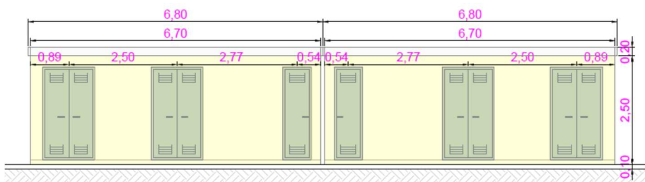
Figura 27: Vista frontale Cabine Prefabbricate
