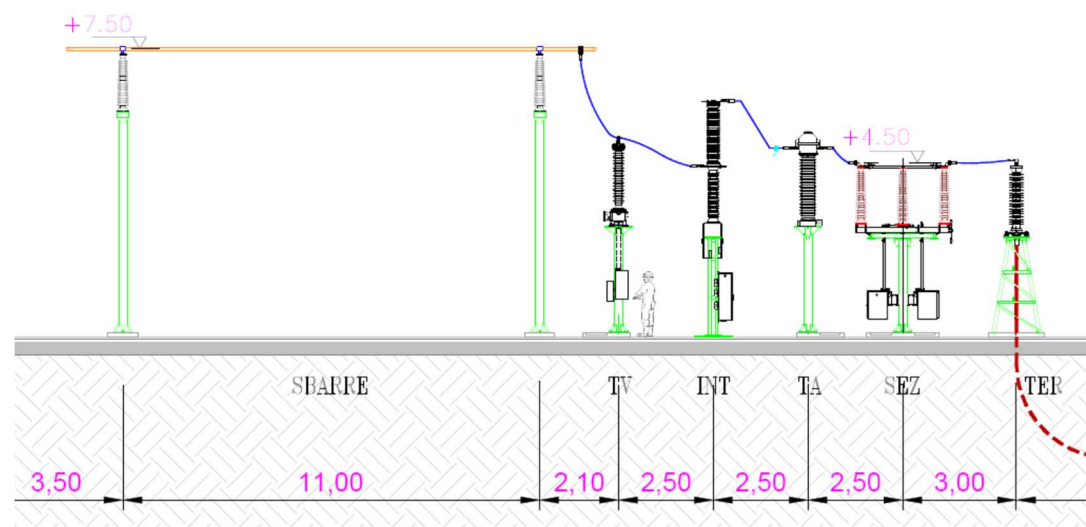
Figura 24: vista prospettica sistema Sbarre Condivise
