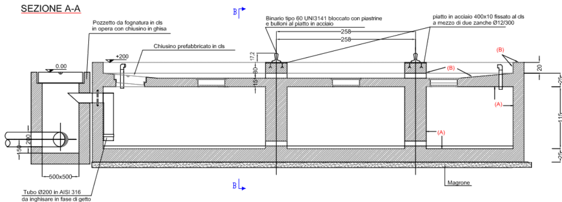
Figura 2: Sezione fondazione trasformatore
