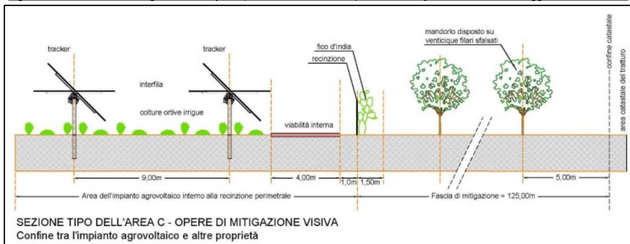
Figura 6.2-C. Fascia di mitigazione di tipo C (Mandorlo-fcodindia) - Area di rispetto Tratturello Foggia-Sannicandro.
