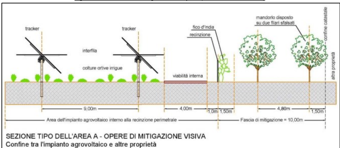
Figura 6.2-A. Fascia di mitigazione di tipo A (Mandorlo-ficodindia)
