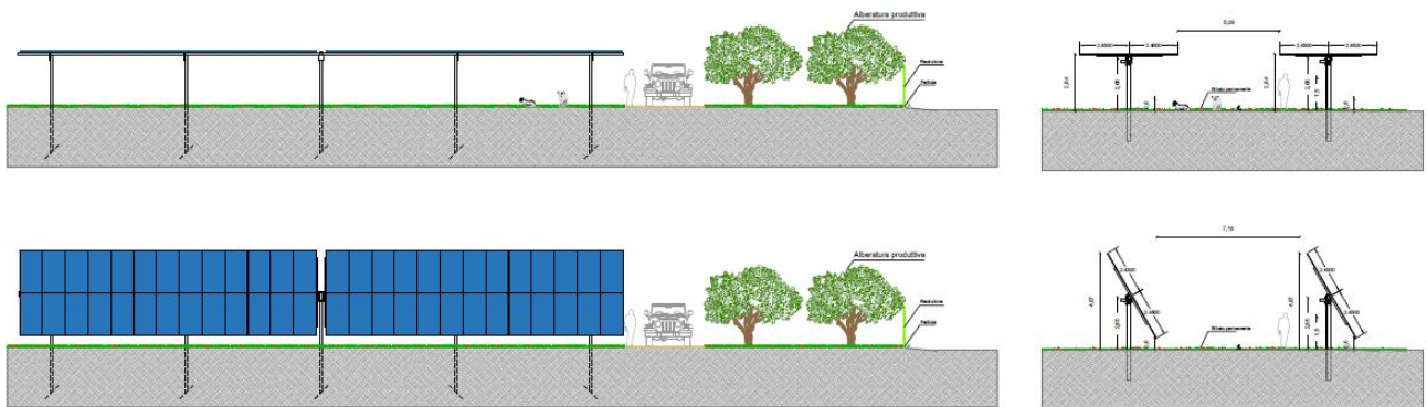
Figura 4 – Sezione significativa del sistema di mitigazione perimetrale.
