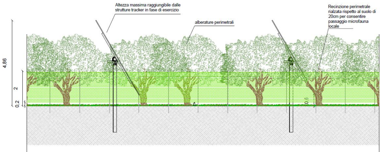
Figura 5 – rappresentazione recinzione perimetrale rialzata dal suolo di 20cm.
