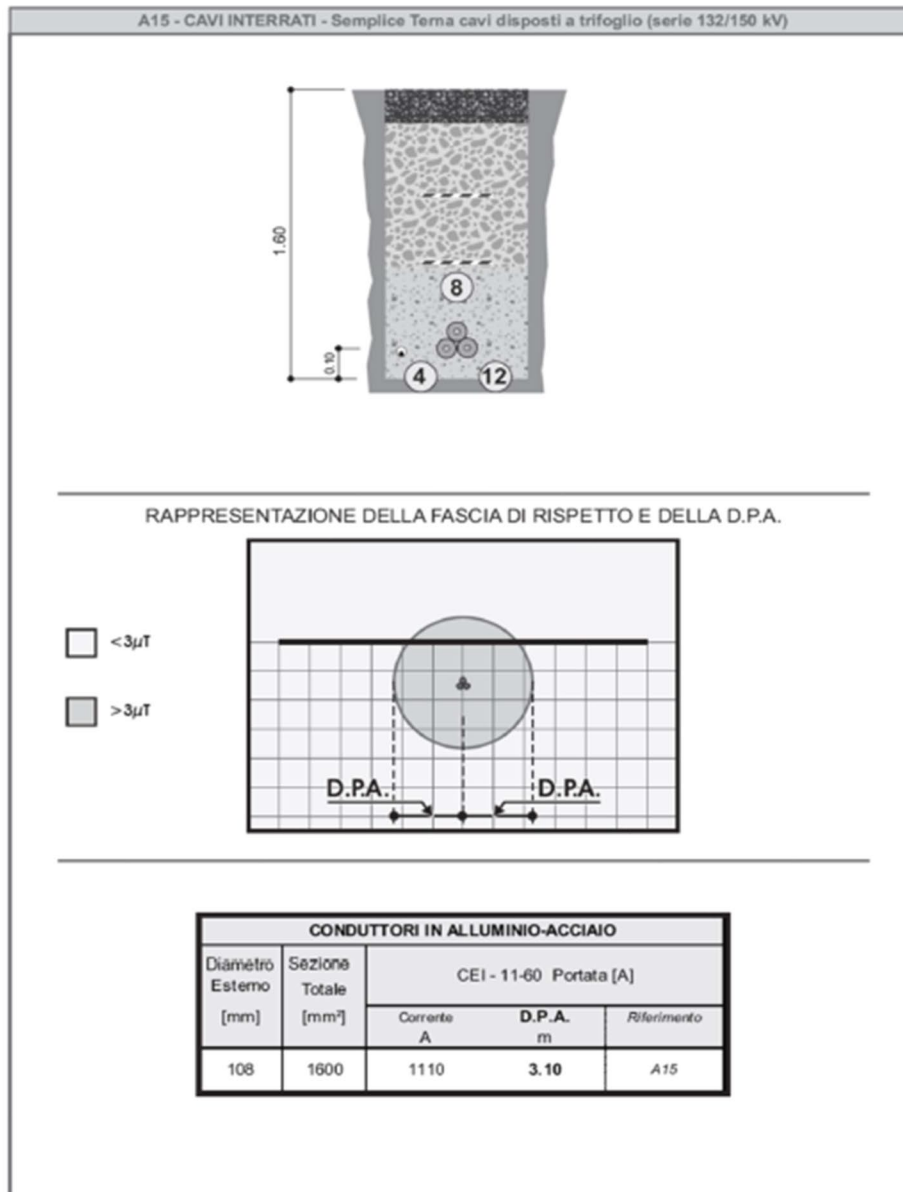
Figura 3: distanza di prima approssimazione linea elettrica AT 150 kV in cavo interrato
