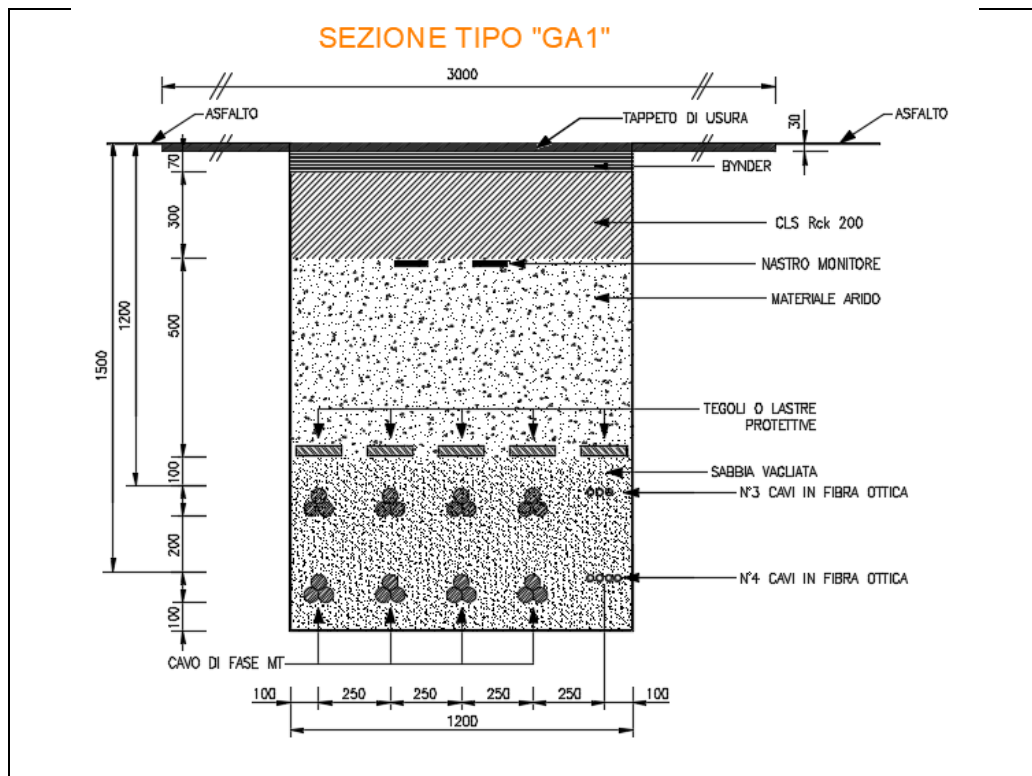
Figura 76: Tipici di posa cavi MT con n°8 linee
