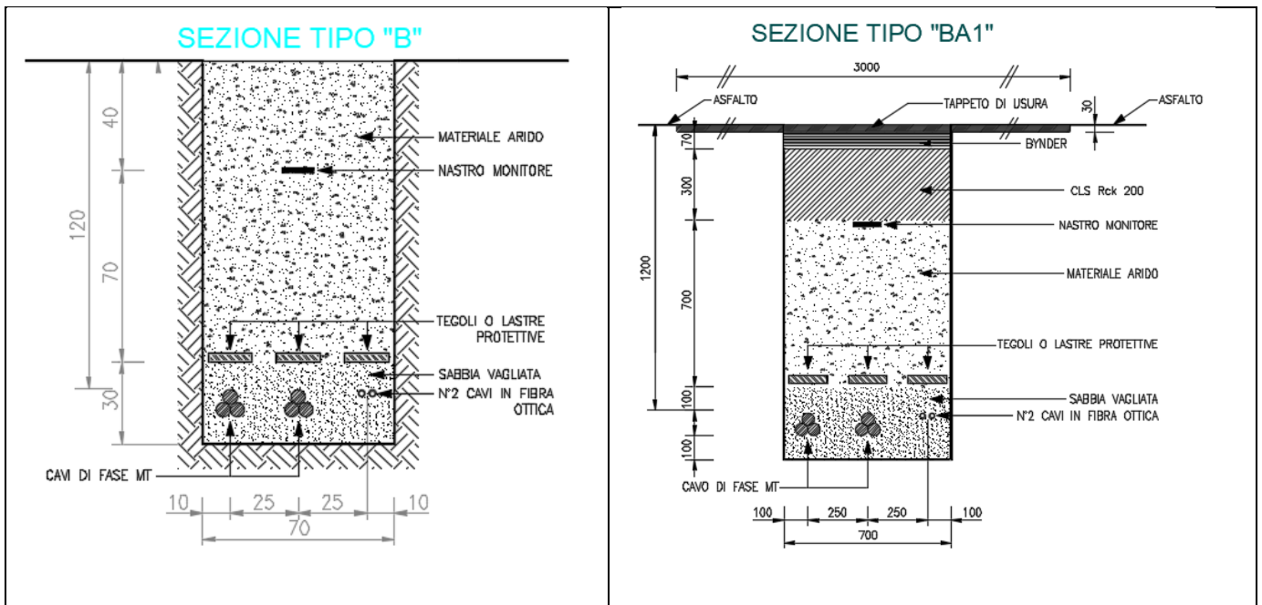
Figura 4: Tipici di posa cavi MT con n°2 linee
