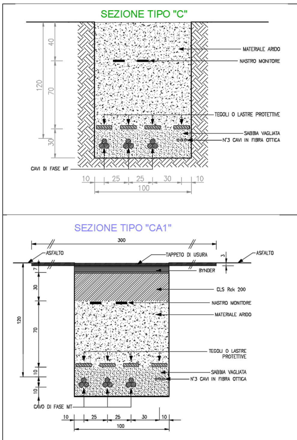
Figura 5: Tipici di posa cavi MT con n°3 linee
