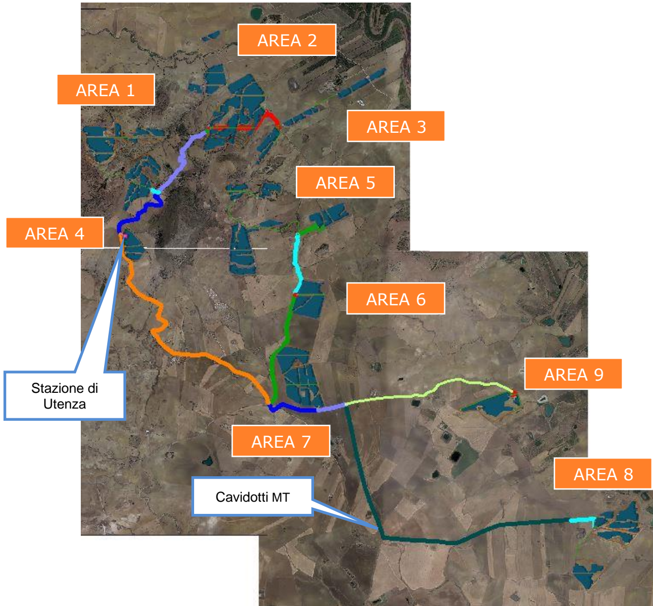
Figura 1: Tracciato degli elettrodotti MT
