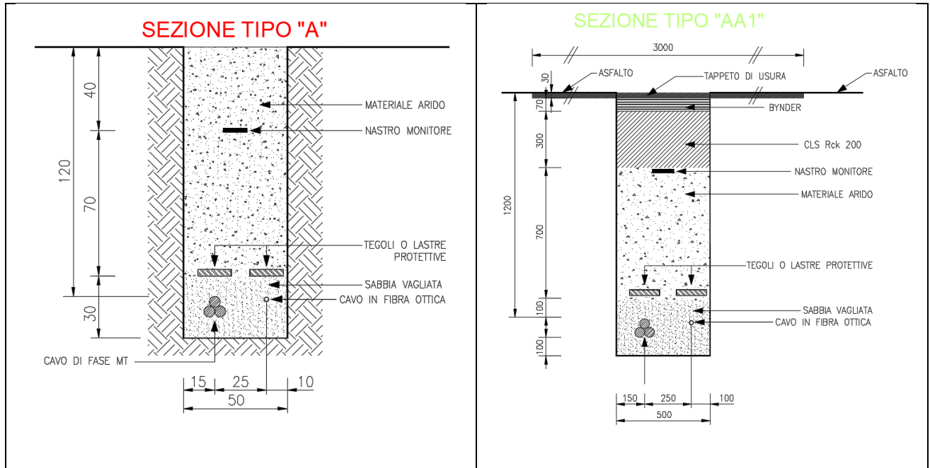
Figura 3: Tipici di posa cavi MT con n°1 linea
